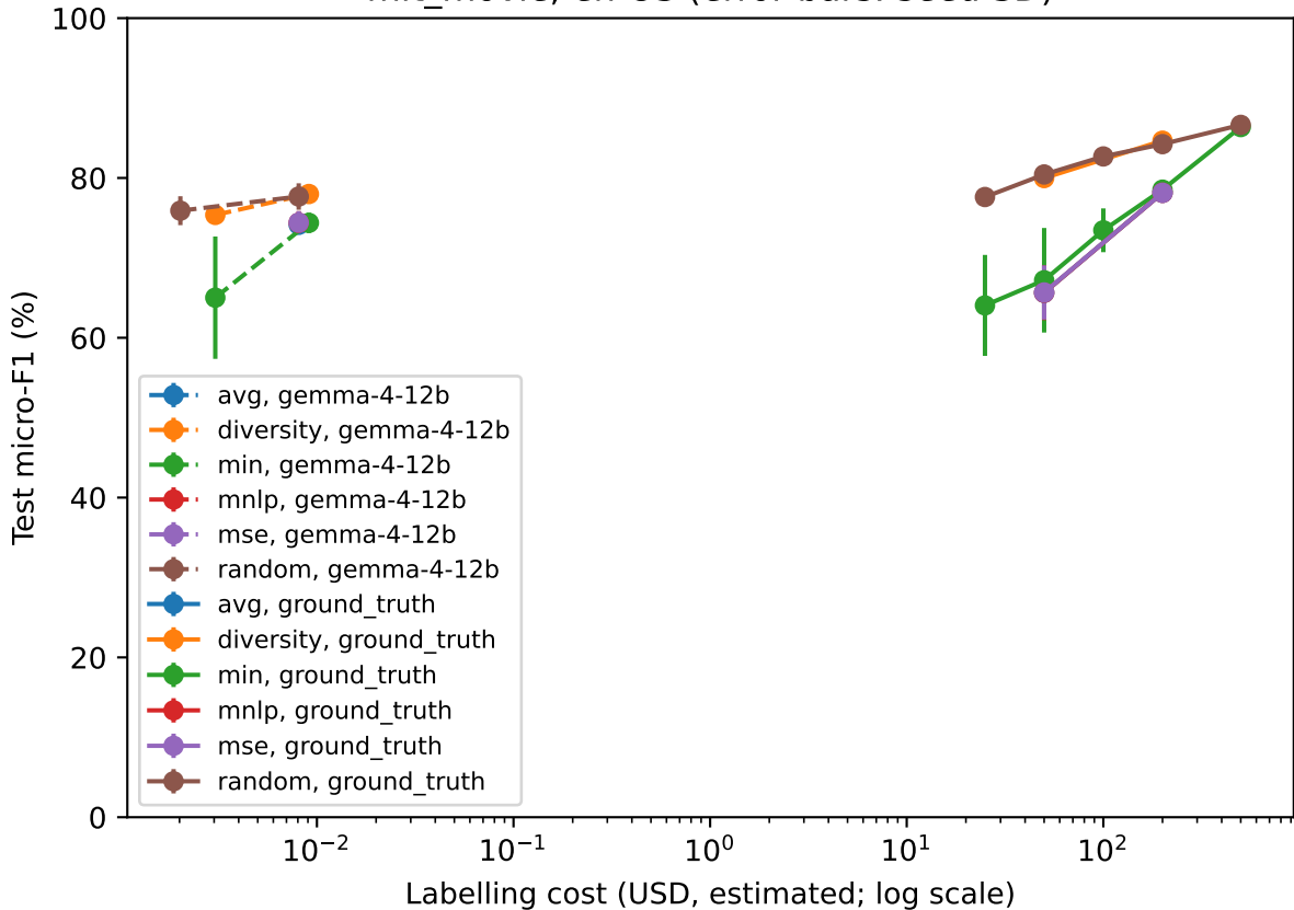
mit movie, en-US (error bars: seed SD)
