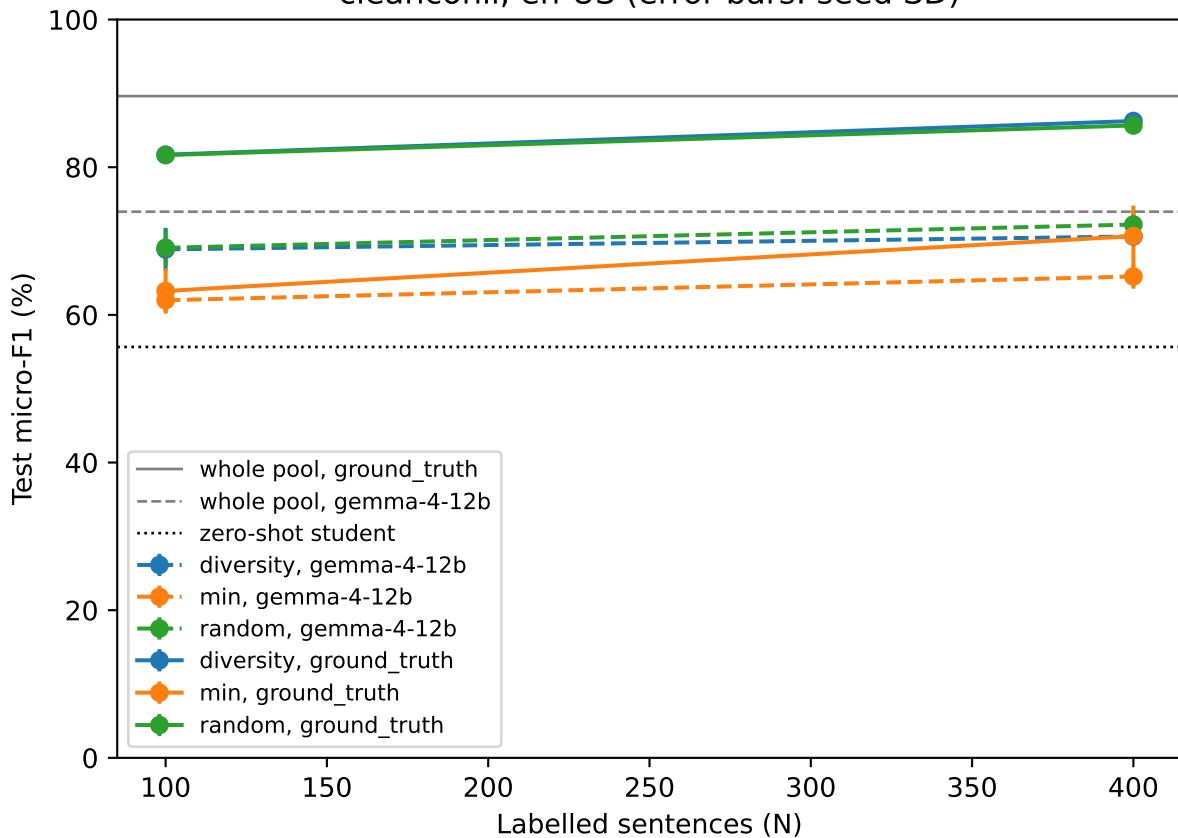
cleanconll, en-US (error bars: seed SD)
