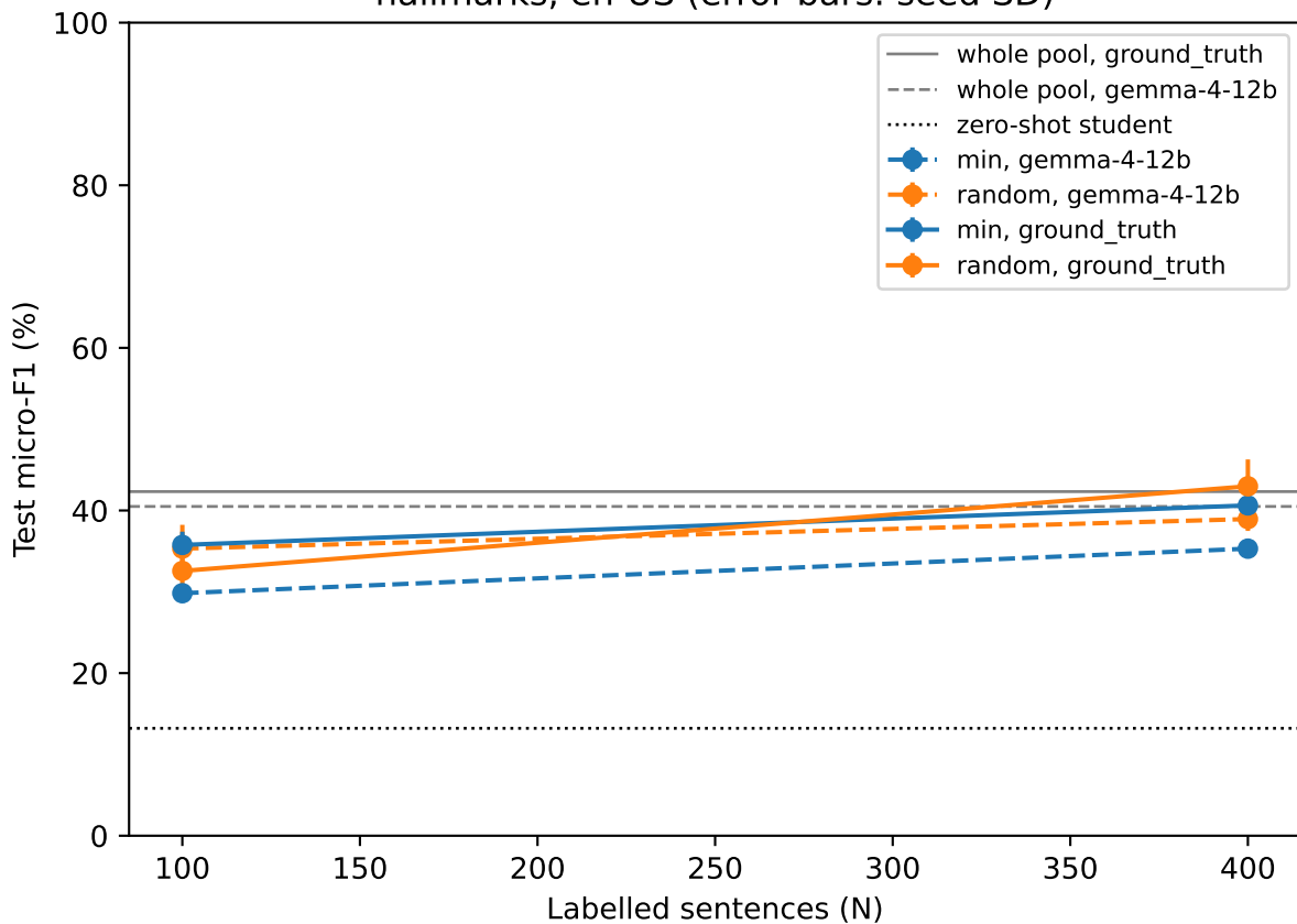
hallmarks, en-US (error bars: seed SD)
