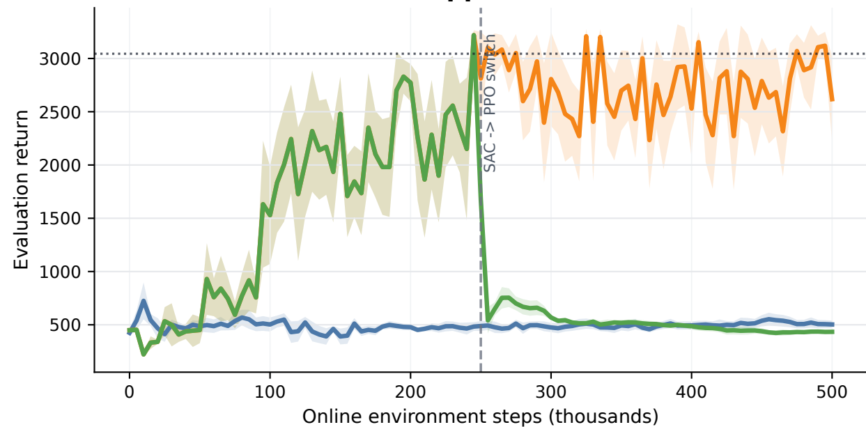
Hopper-v4
