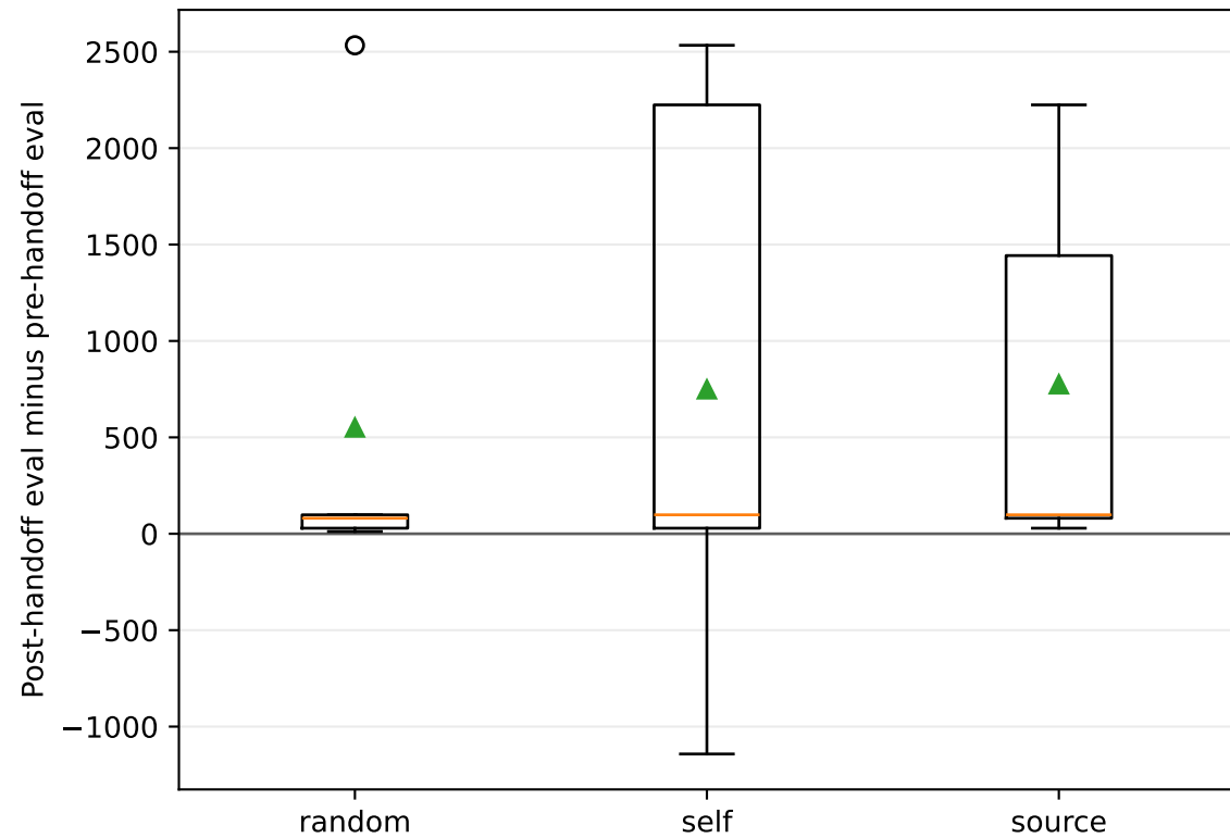
Hopper-v4
