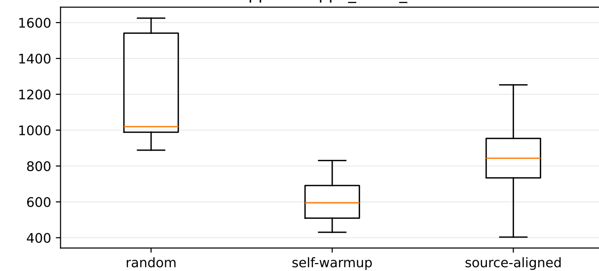
Hopper-v4: ppo_value_loss
