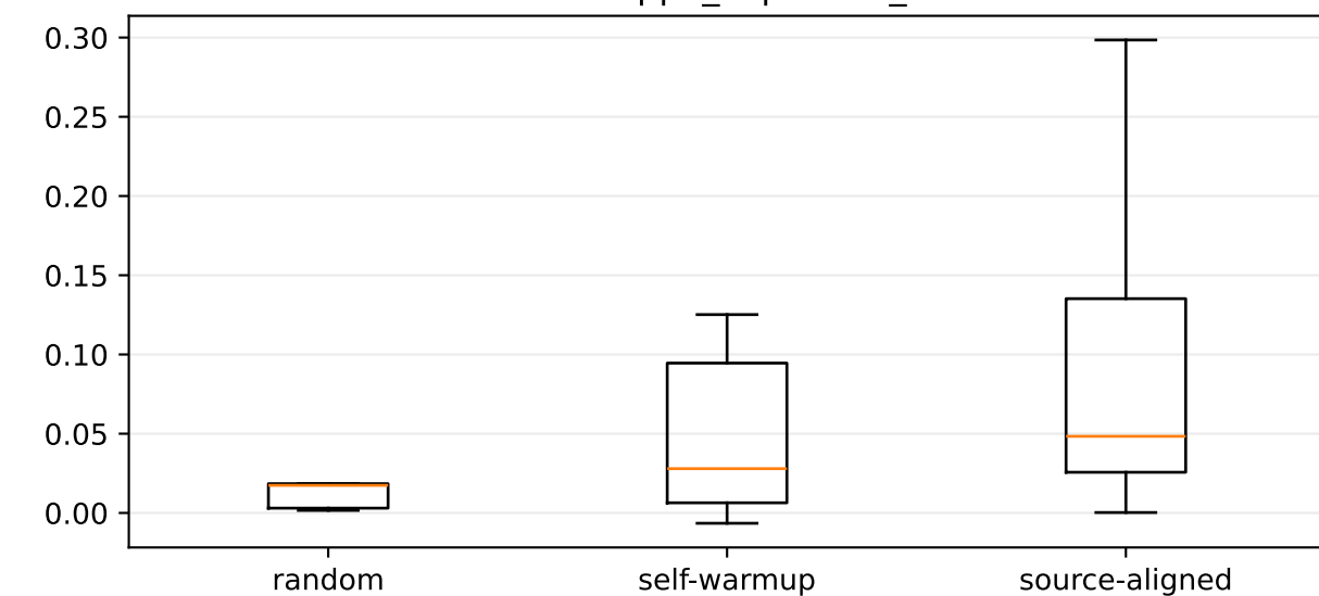
Walker2d-v4: ppo_value_loss
