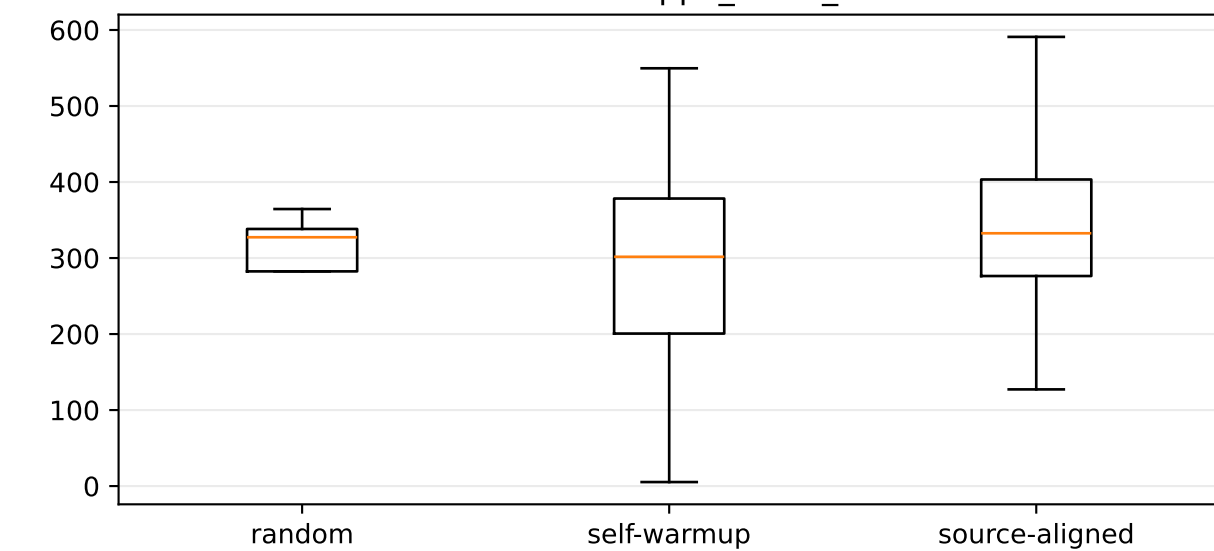
Walker2d-v4: ppo_value_loss
