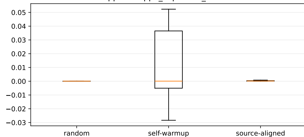
Hopper-v4: ppo_value_loss
