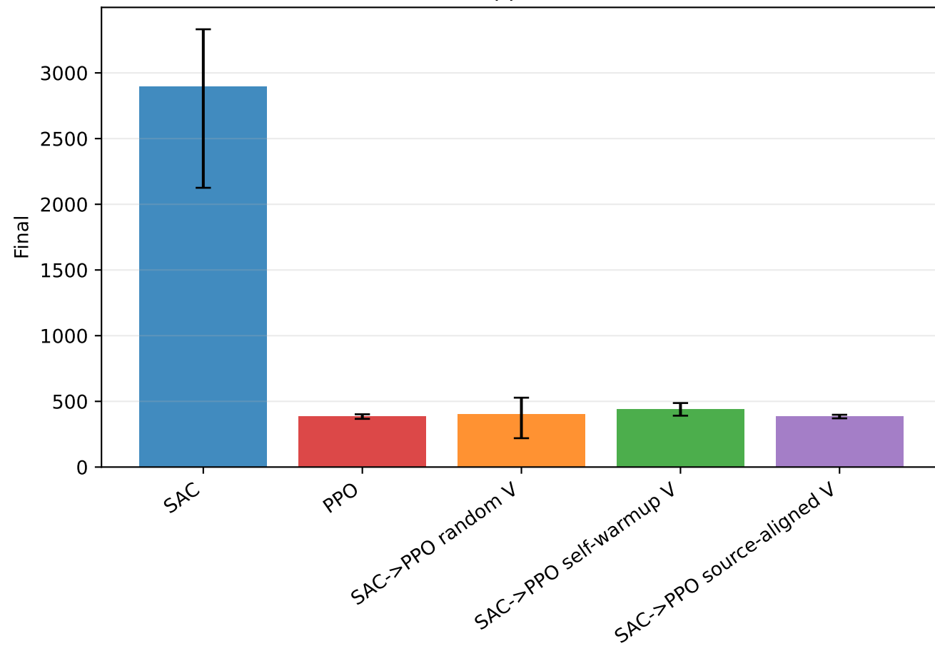
Hopper-v4
