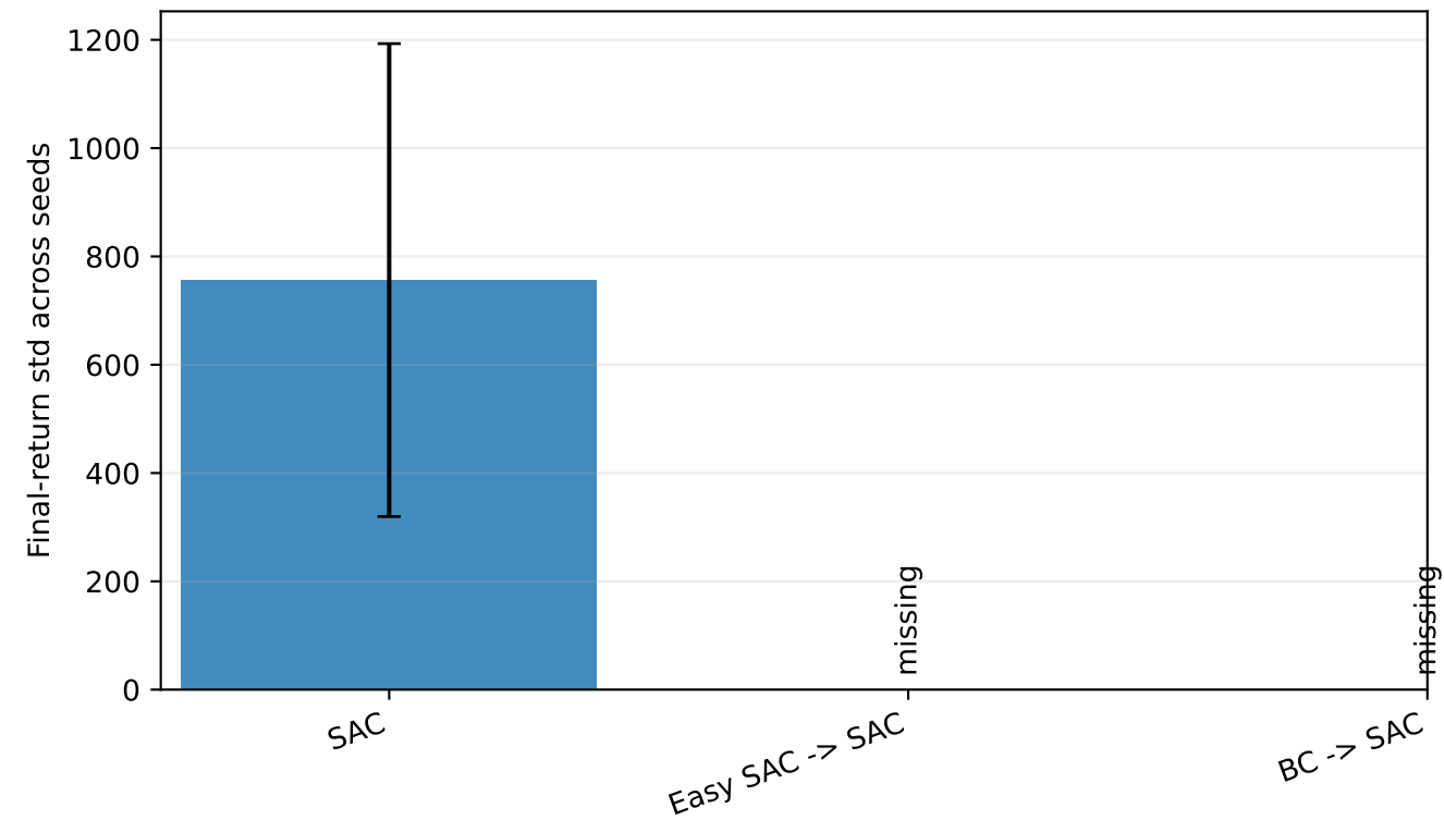
Ant-v4
