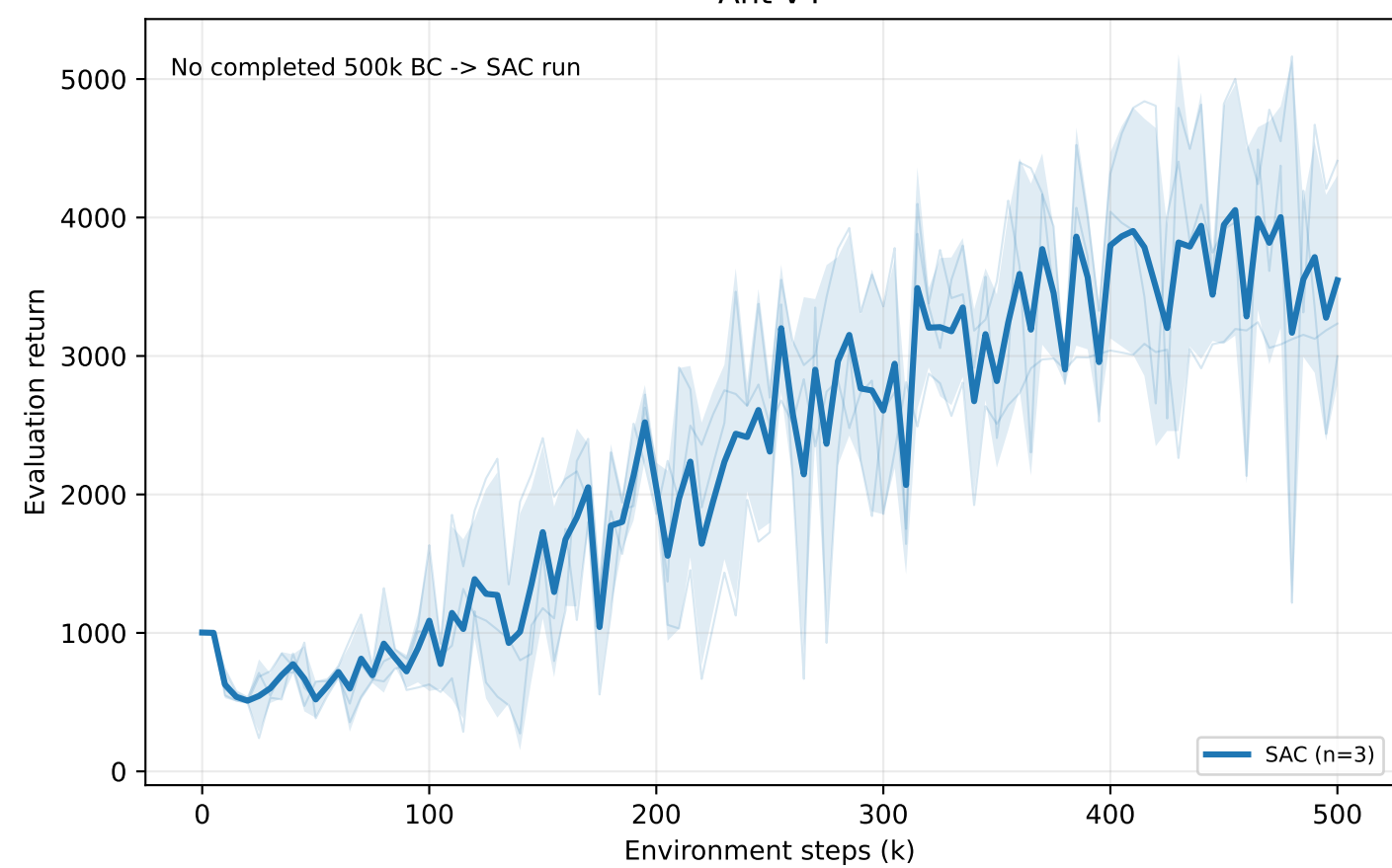
Ant-v4
