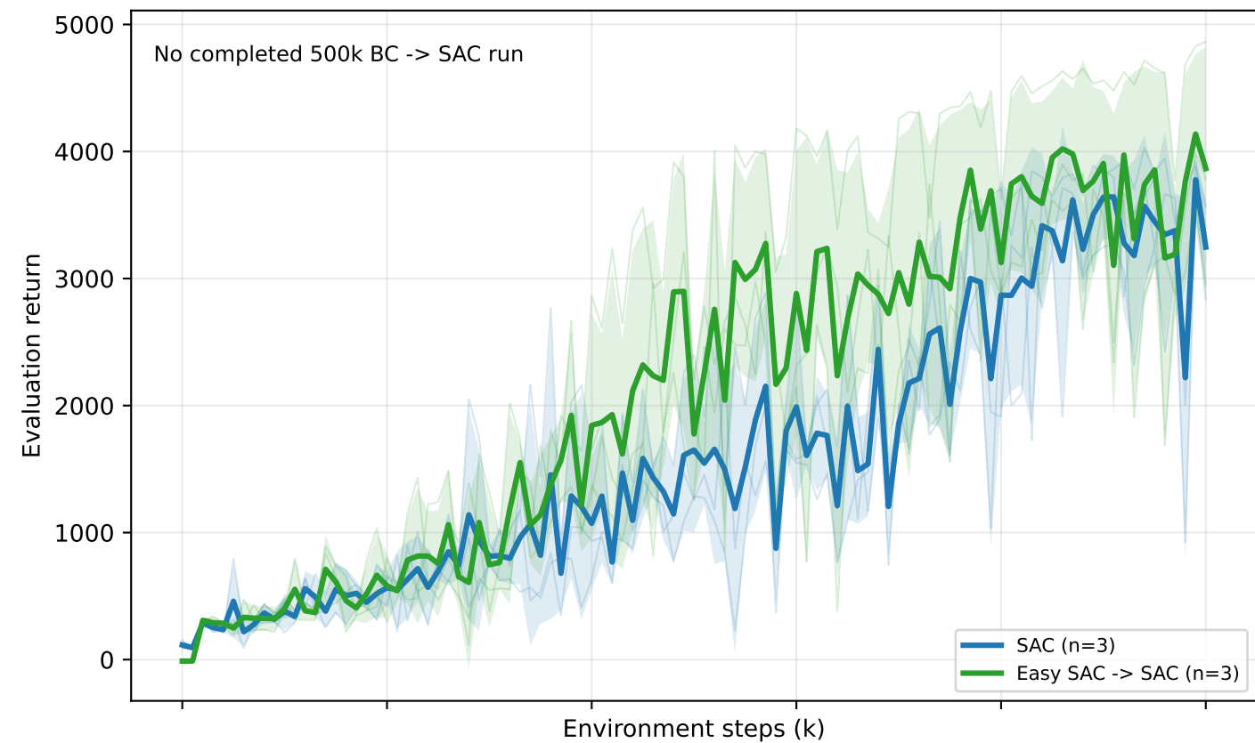
Ant-v4
