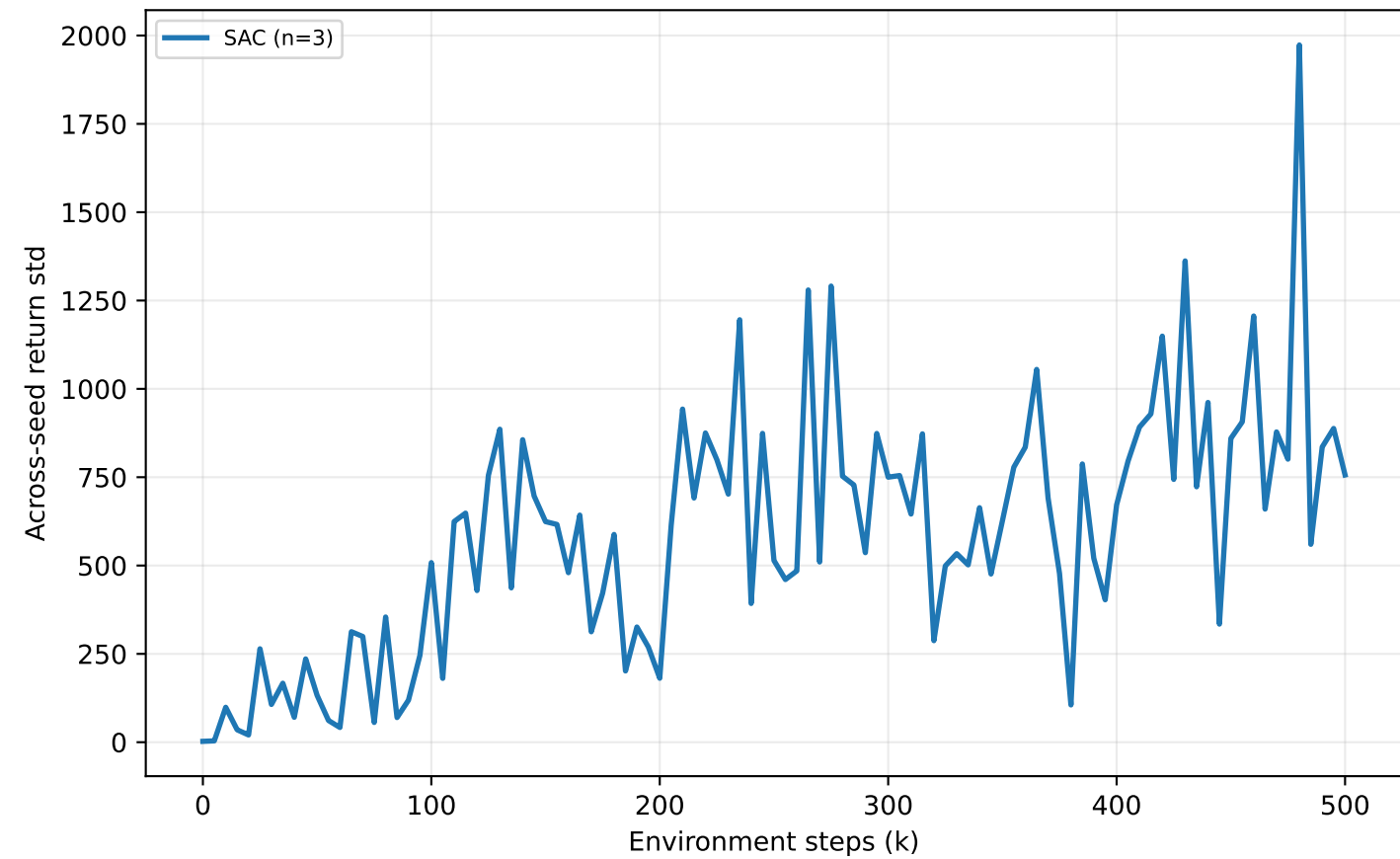
Ant-v4
