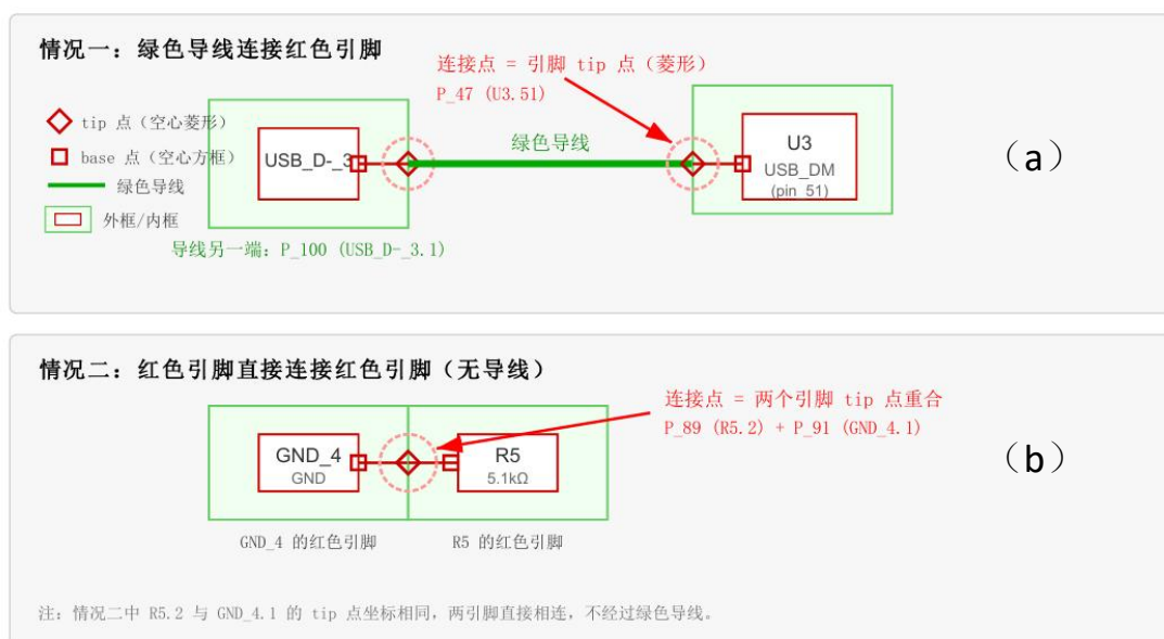
图八：引脚连接方式示意图
