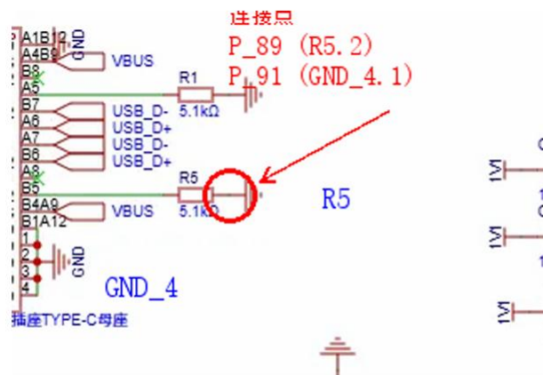
图十：引脚连接示意图
