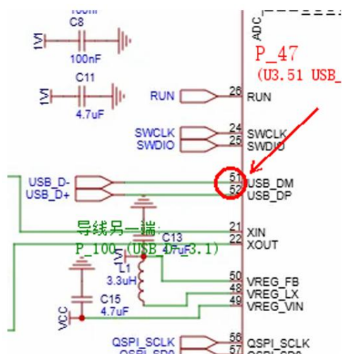
图九：引脚连接示意图
