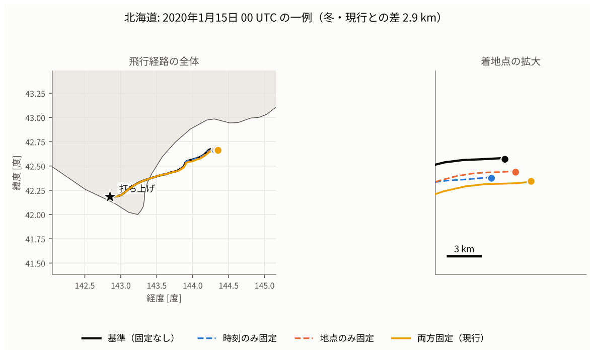
図 70: 2020 年 1 月 15 日 00 UTC に VOISING から上げた場合の飛行経路。左が全体、右が着地点の拡大。この例では 4 通りの差が 2.9km しかなく、和歌山の同じ日 (図 68、13.1 km) よりずっと小さい。和歌山では基準 (黒) と時刻のみ固定 (青)、地点のみ固定 (橙) と両方固定 (黄) がそれぞれ対になるのに対し、ここでは 4 本が順に並ぶだけで、そうした対応は見えない。1 例は 1 例であって統計ではない。どちらが典型かは表 22 で判断してほしい。
