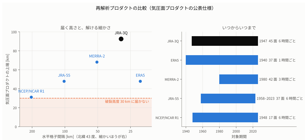
図 1: 主な再解析の比較。左は横軸が水平格子間隔（細かいほうが右）、縦軸が気圧面プロダクトの上端高度。本用途に適するのは右上で、下の帯は破裂高度 30 km に届かない範囲である。右は対象期間と、気圧面の数・解析間隔。 JRA-3Q の値だけが実測で、本パイプラインが取得したファイルから読んでいる。他は各提供元が公表している気圧面プロダクトの仕様を手で入力したもので、モデル格子やモデル面の仕様ではない。仕様は更新されうるので、自分の研究に選ぶときは最新の値を確認してほしい。
