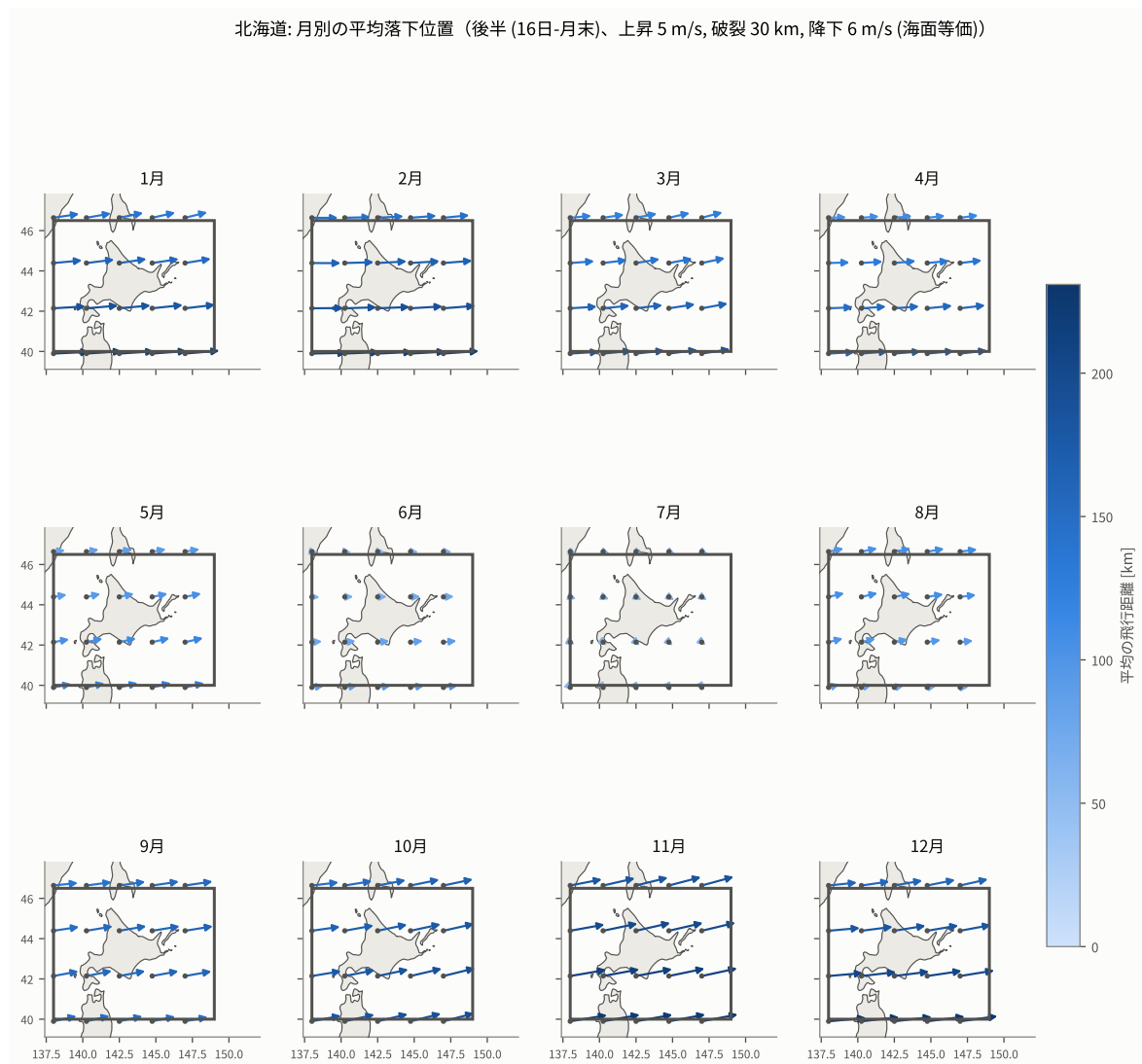
図 25: 各格子点から上げた場合の平均落下位置。矢印は実寸で、矢先がそのまま予測落下点である。色が平均の飛行距離。全パネルが同じ枠と同じ色スケールなので、月どうしを直接比べられる。
