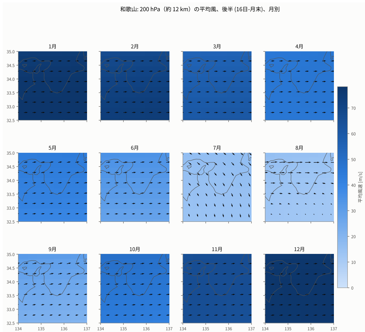
図 40: 200 hPa (約 12 km) の平均風を月ごとに並べたもの。塗りが風速、矢印が風向。ジェットが季節とともに動く様子が地図の上で見える。
