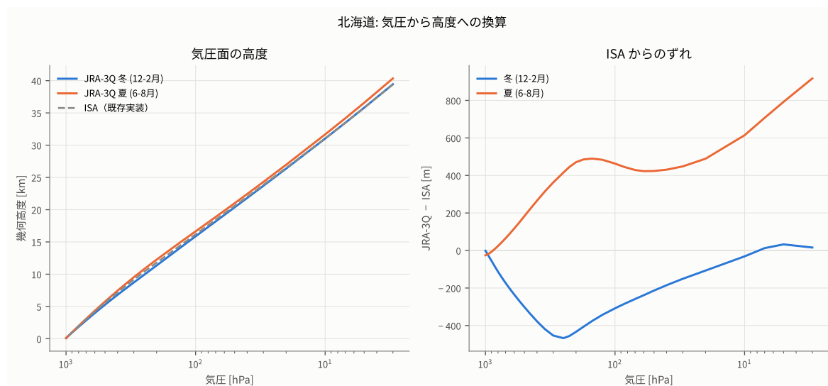
図 32: 気圧から高度への換算。左は JRA-3Q の実際の気圧面高度と、既存シミュレータが使う国際標準大気 ISA。右はその差。ISA は季節も緯度も天気も知らないので、季節によって系統的にずれる。
