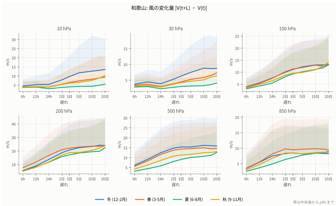
図 56: 遅れ L を置いたときの風の変化量 |V(t+L) - V(t)| 。実線が中央値、帯が p90 まで。横軸は対数で、6 時間から 20 日まで。組は両端が同じ季節に入るものだけを数えている。10 hPa と 30 hPa の曲線が遅れ 24 時間でいったん下がるのは大気潮汐による見かけの効果である。
