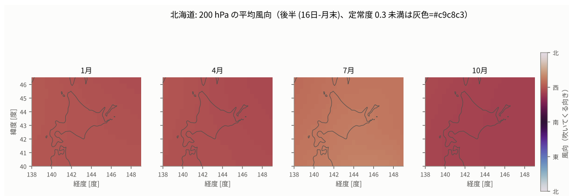
図 22: 200 hPa の平均風向。円環用のカラーマップを使い、定常度 0.3 未満は灰色にしている。灰色の領域では平均風向に意味がない。
