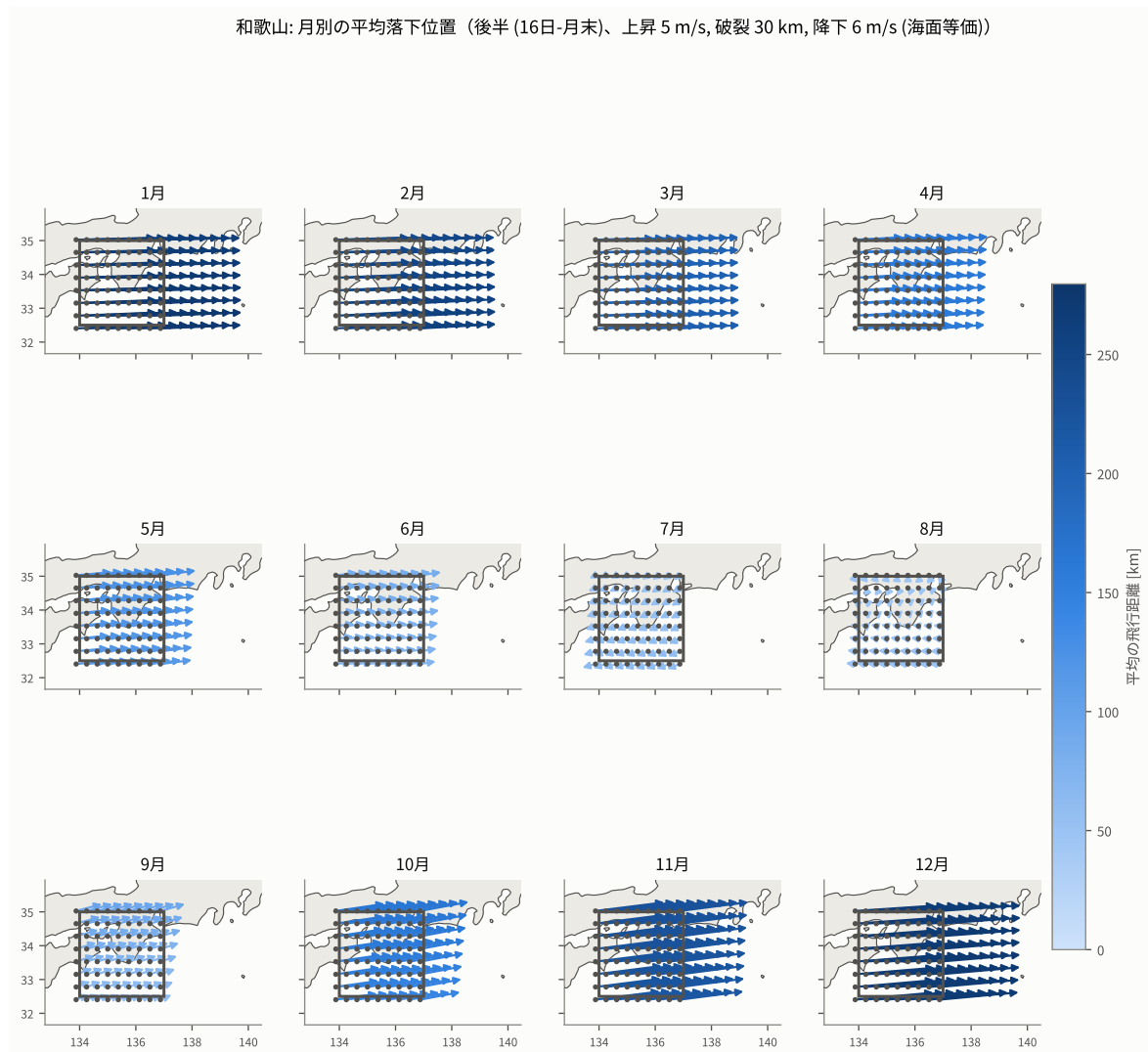
図 45: 各格子点から上げた場合の平均落下位置。矢印は実寸で、矢先がそのまま予測落下点である。色が平均の飛行距離。全パネルが同じ枠と同じ色スケールなので、月どうしを直接比べられる。
