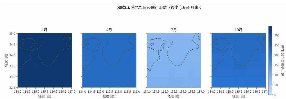
図 48: 飛行距離の 90 パーセントイル。平均 150 km で p90 が 400 km という状況と、平均 150 km だけを見て計画することは、運用上まったく違う。
