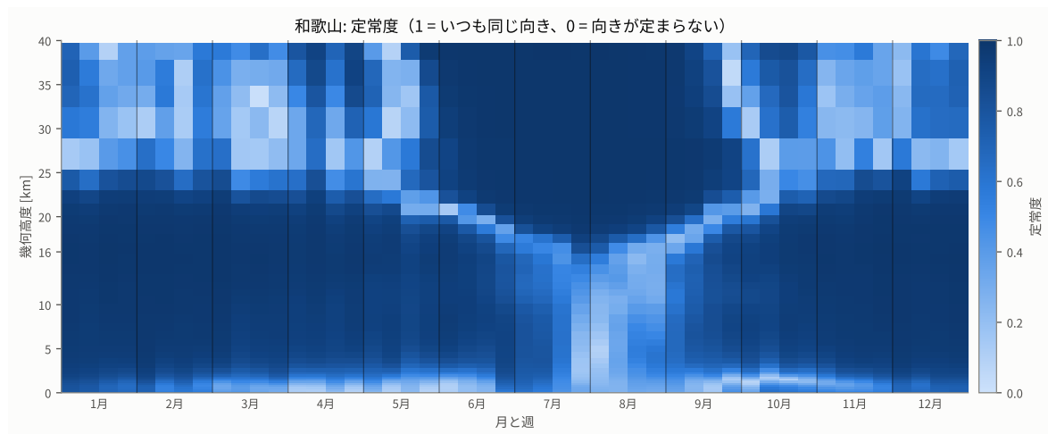
図 36: 定常度 (ベクトル平均風速 ÷ スカラー平均風速)。1 に近いほど風向が安定し、0 に近いほどピンのかで風向が入れ替わっている。淡い帯が成層圏の風の反転している高度で、季節とともに上下する。
