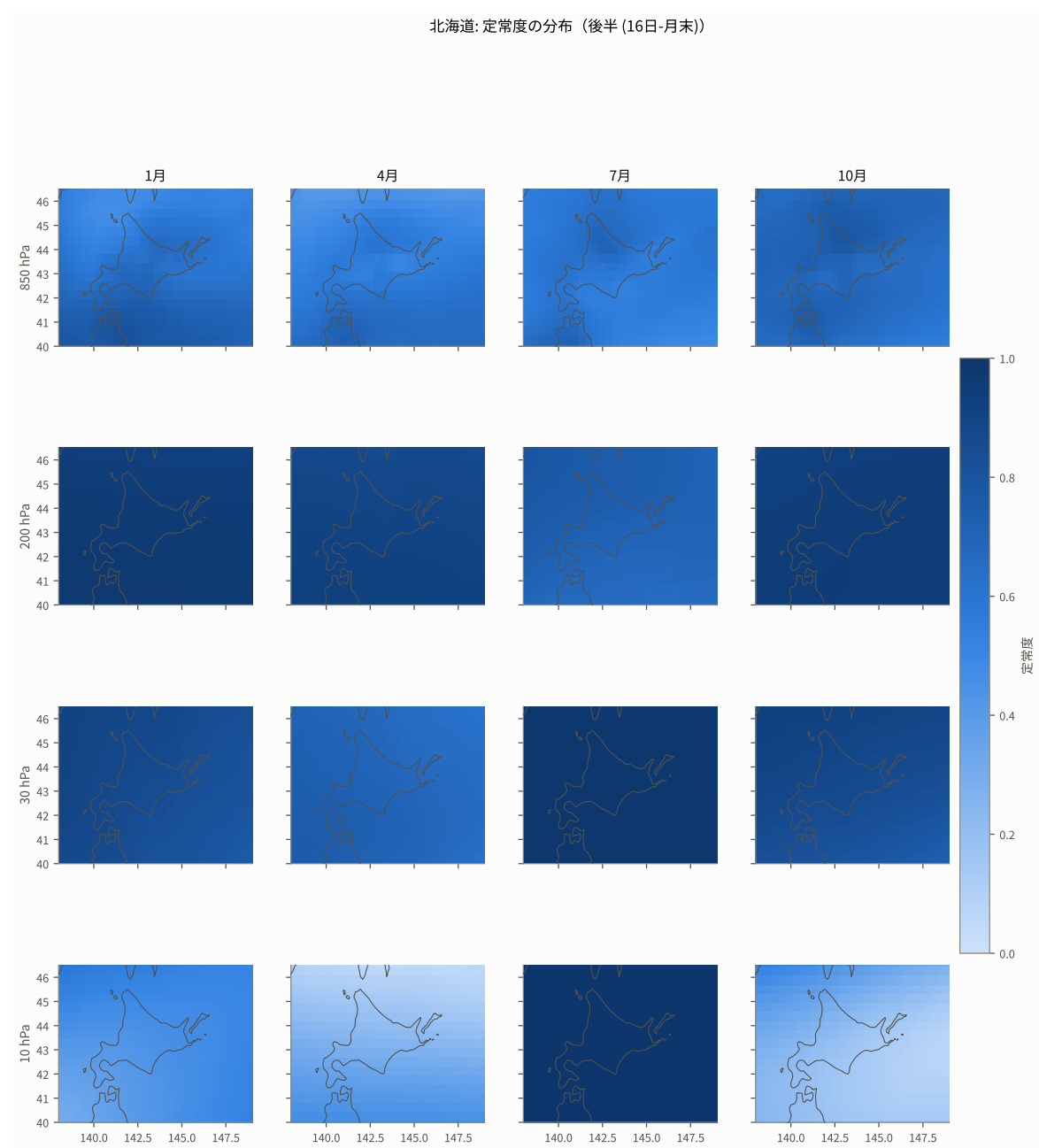
図 23: 高度と季節ごとの定常度。濃いところでは風向が安定していて計画が立てやすく、淡いところではビンのなかで風向が入れ替わる。
