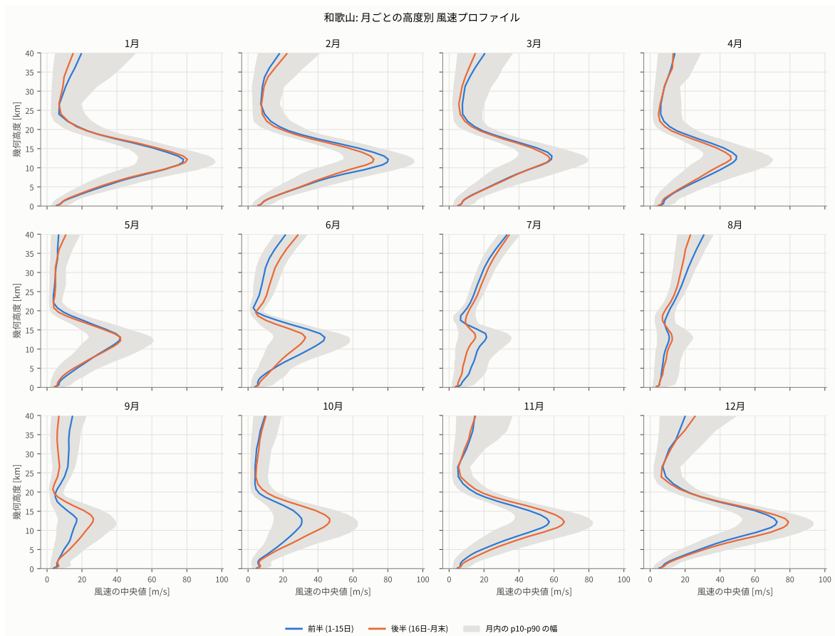
図 35: 月ごとの風速プロファイル。線は各ビンの中央値、灰色の帯はその月の 2 ビンを通した p10-p90 の広がり。帯の幅が「ふつうからのずれ方」であり、線だけを見て計画を立ててはいけない。
