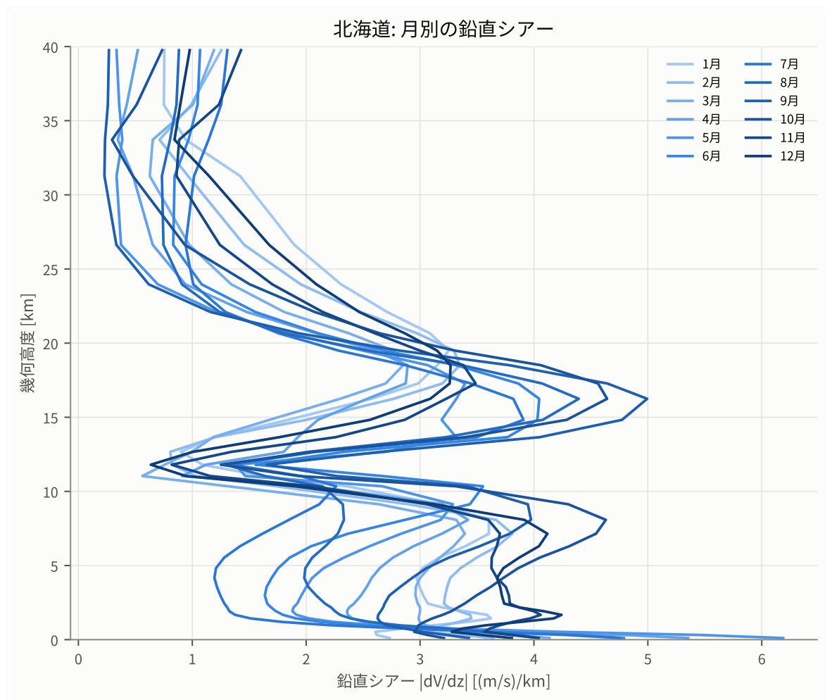
図 31: 隣り合う気圧面のあいだの風速差を高度差で割ったもの。気球そのものはシアーで壊れないが、大きいところでは高度の推定が少しずれるだけで水平の予測が大きく動く。最大はジェットの下と地表付近に出る。
