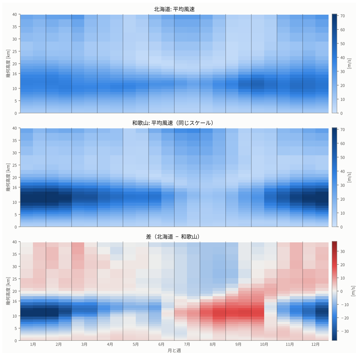
図 55: 上 2 段は同じカラースケールでの平均風速、下段はその差（北海道－和歌山）。赤は北海道のほうが強いピン・高度、青は和歌山のほうが強いピン・高度である。
