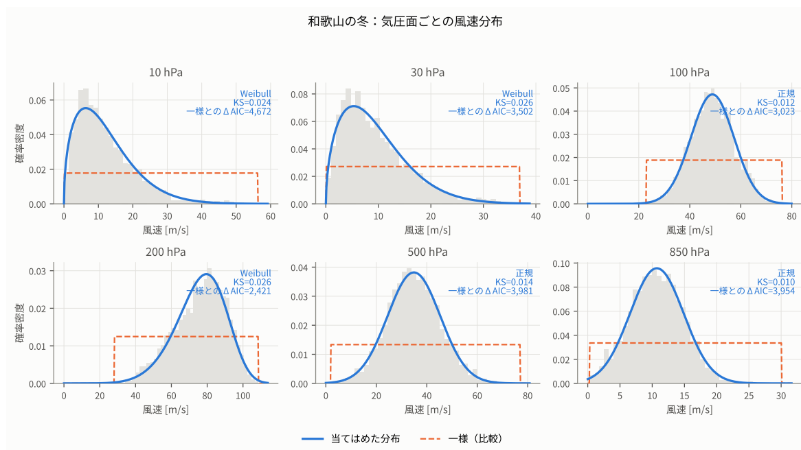
図 72: 和歌山の冬、代表的な 6 つの気圧面での風速のヒストグラムと、当てはめた分布（青）。比較のため一様分布（橙の破線）も重ねてある。採用した分布の名前・KS 統計量・一様分布との \Delta AIC を各パネルに記した。採用した分布が面によって正規と Weibull に分かれるので、凡例ではなくパネルごとに名前を書いている。
