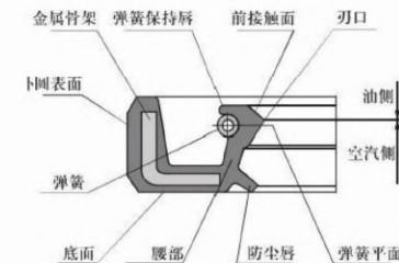
普通标准型产品断面
