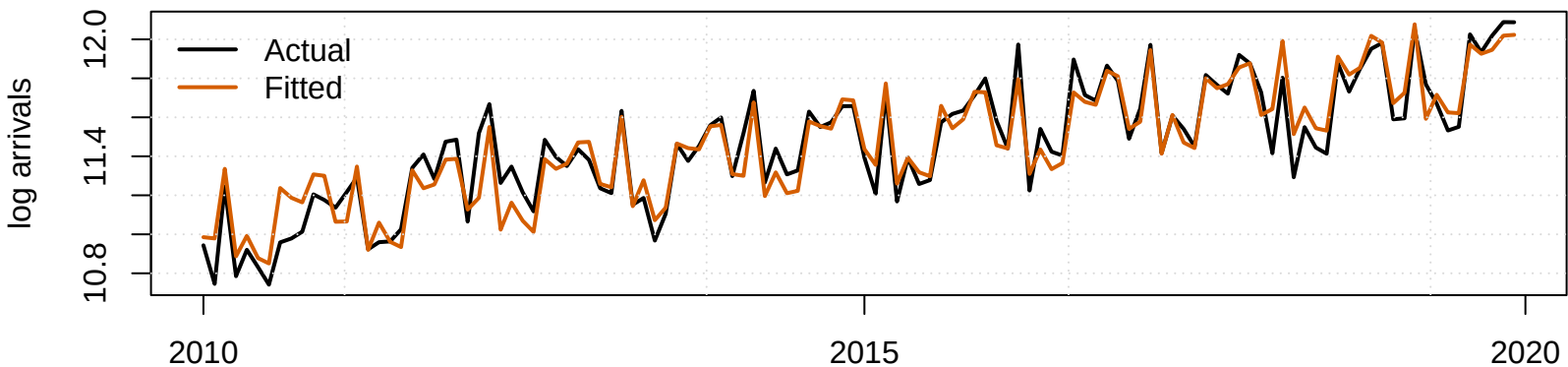
Actual vs fitted values: Model 01
