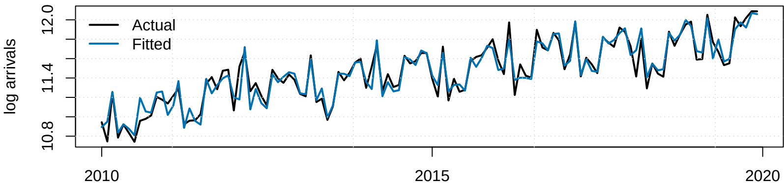
Actual vs fitted values: Model 02
