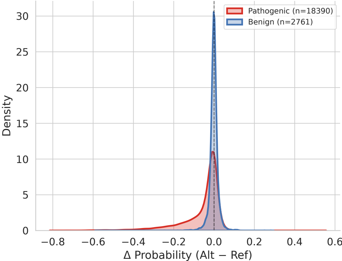
ORF
