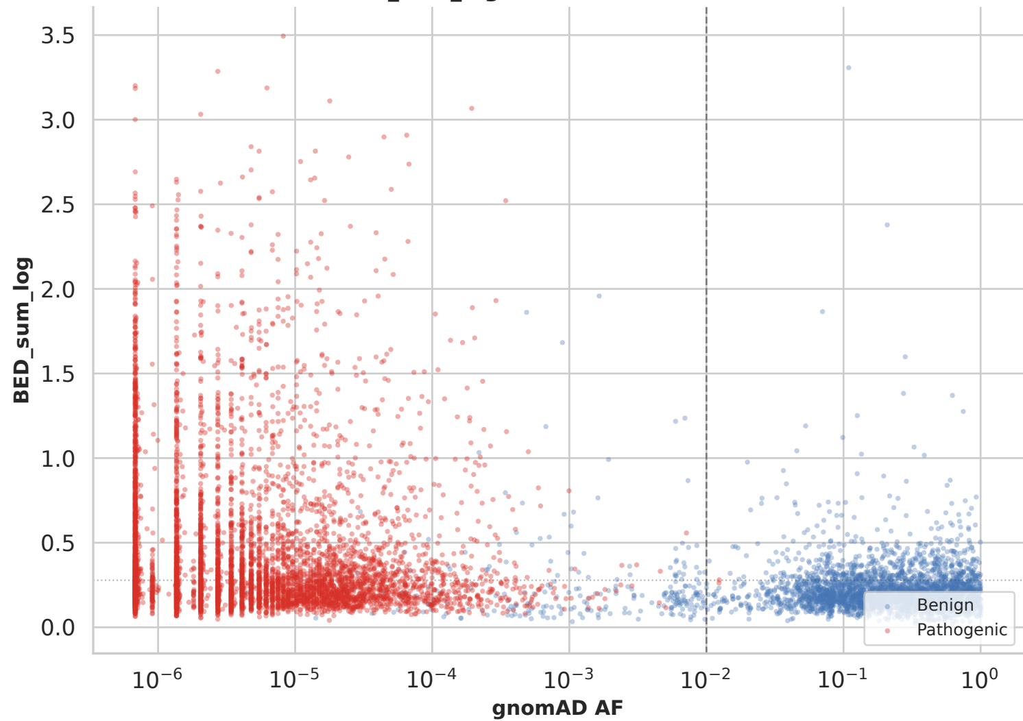
BED_sum_log (AUC=0.673, d=0.57)
