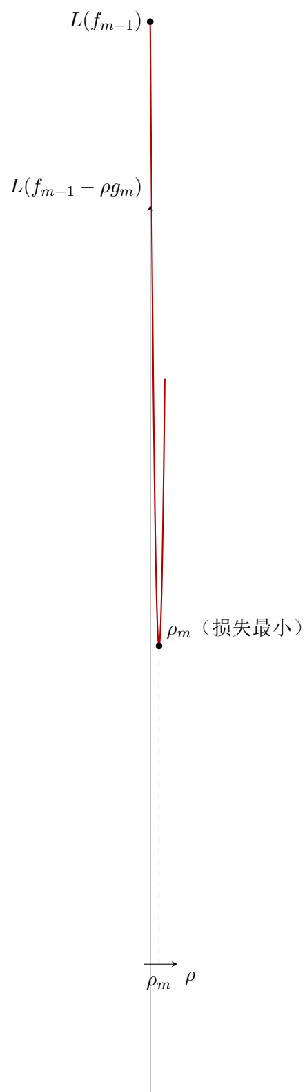
图 (剖面视角): 沿 -g_m 方向的损失 L(f_{m-1} - \rho g_m) 随 \rho 变化: 先降后升, 谷底 \rho_m 处损失最小——即相对旧点 f_{m-1} 的损失下降量在该方向上最大。
