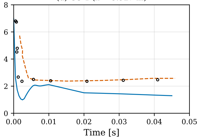
(d) GS-1 ( x = 3.927 m)
