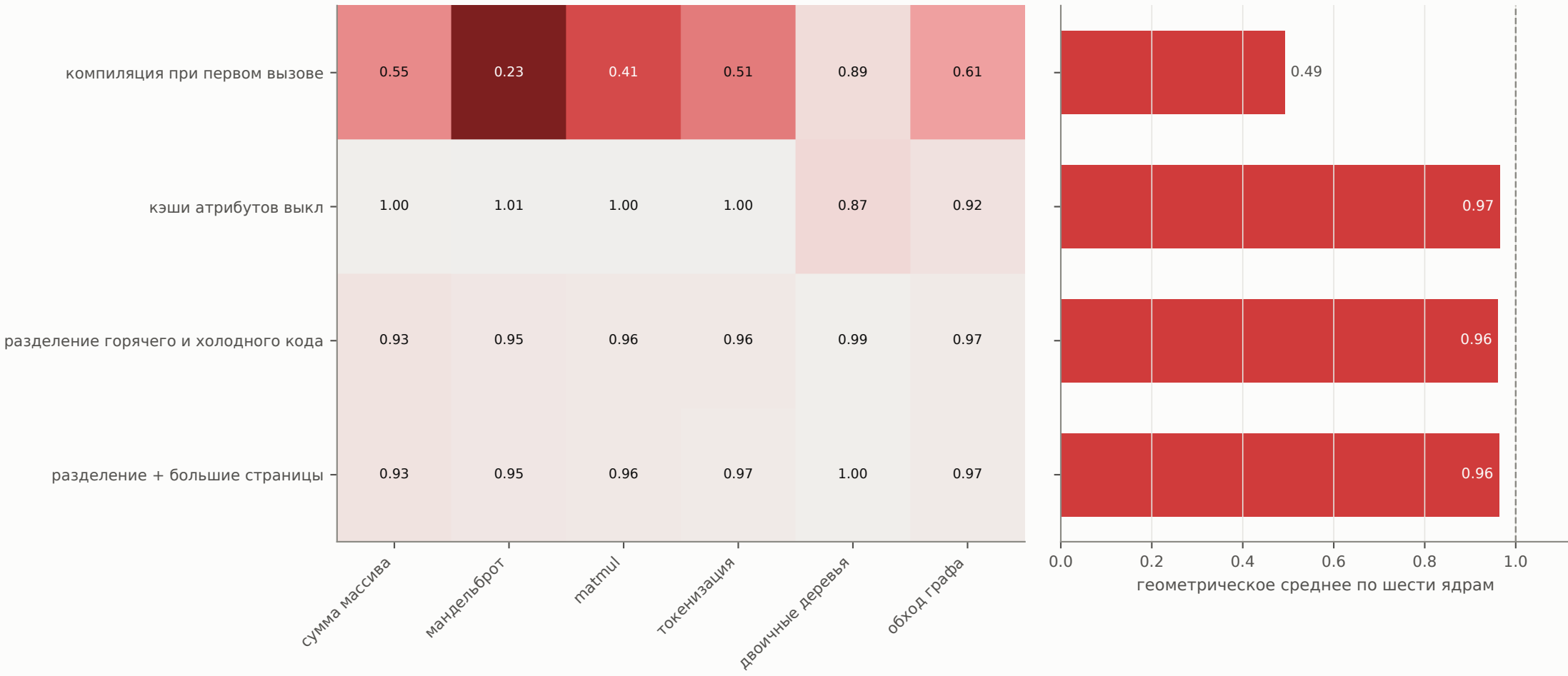
Скорость относительно конфигурации JIT по умолчанию (>1 — быстрее)
