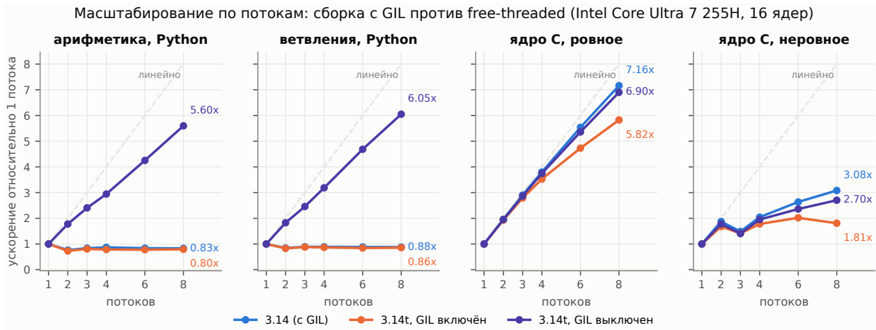
Рис. 10: B5: масштабирование по потокам. Ускорение приведено относительно той же конфигурации на одном потоке, пунктир — линейное масштабирование.
