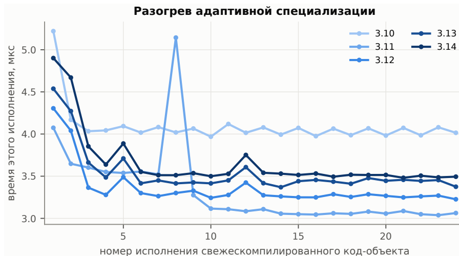
Рис. 7: ВЗ: время одного исполнения свежекомпилированного код-объекта на первых его исполнениях, по выпускам. Каждая точка — отдельный бенчмарк puregf , измеряемая область которого и есть это одно исполнение.
