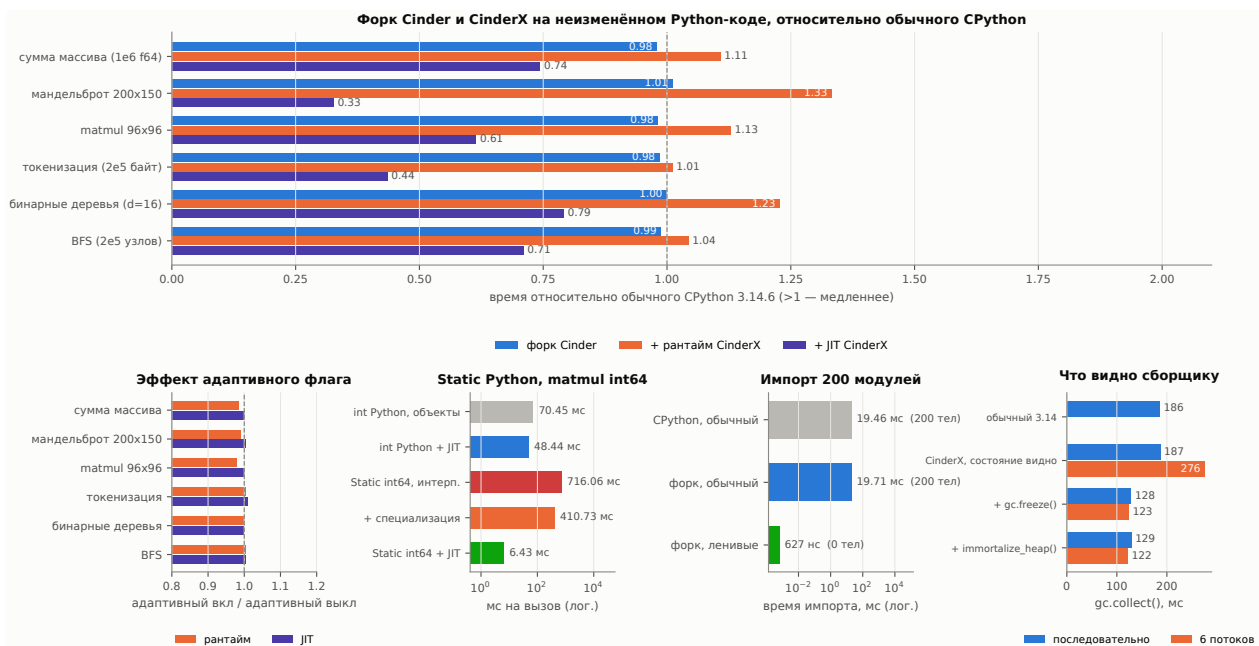
Рис. 8: B4: (сверху) форк, рантайм CinderX и JIT CinderX на неизменённом Python-коде относительно обычного CPython 3.14.6, собранного теми же флагами, (снизу слева) влияние флага адаптивного Static Python на те же отношения, (снизу в центре) целочисленный matmul на Static Python int64 (построено для медленной раскладки, 6.43 мс; быстрая — 4.25 мс, §7) — против того же ядра с объектами и того же ядра с объектами под JIT, а также в интерпретаторе без адаптивной специализации и с ней, (снизу правее центра) задержка импорта пакета из 200 модулей с ленивыми импортами форка и без них, (снизу справа) одна сборка кучи воркера — долгоживущее состояние плюс мусор на запрос — при видимом сборщику состоянии, после gc.freeze() и после immortalize_heap() , последовательно и на шести потоках, с обычным CPython на той же куче для сравнения.
