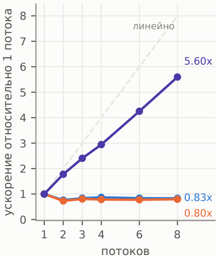
арифметика, Python
