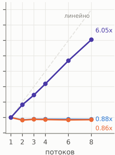
ветвления, Python
