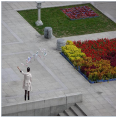
input (192×192)
