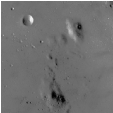
input (192×192)
