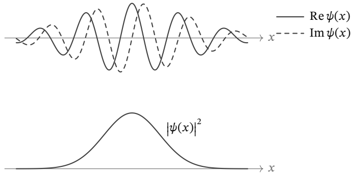
Gambar 1: Grafik fungsi gelombang \psi(x) , termasuk bagian real dan imajinernya. Bagian bawah gambar menunjukkan kerapatan probabilitas |\psi(x)|^2 . Luas total di bawah kurva adalah 1.
