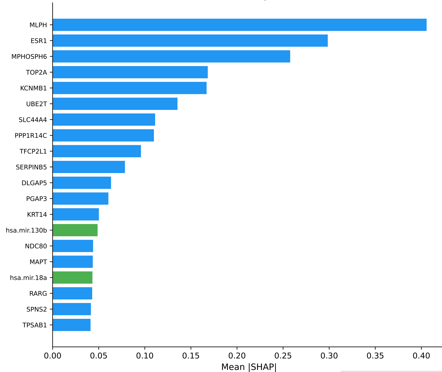
XGBoost SHAP Top 20 -- BRCA
