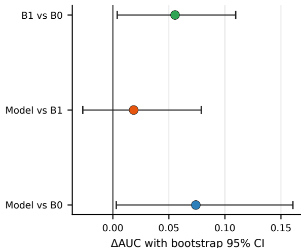
B. Incremental AUC
