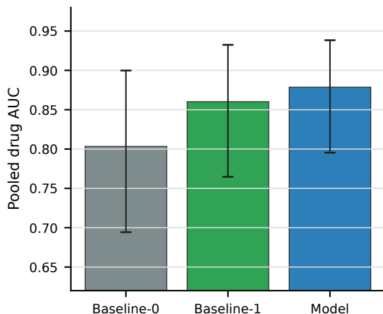
A. Leave-one-out AUC
