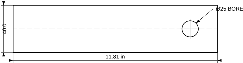
SHAFT - LONGITUDINAL VIEW
