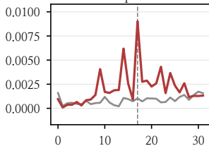
Llama
