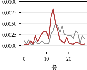
Llama
