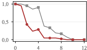
Llama
