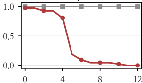
DeepSeek
