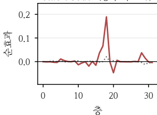
StableCode (봉우리 L18)
