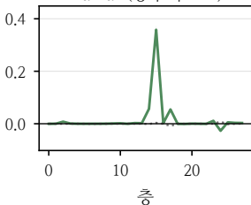
Llama (봉우리 L15)
