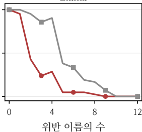
Llama
