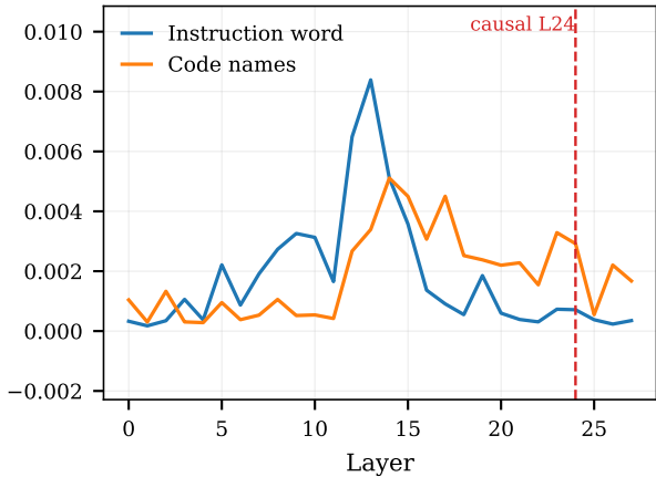
Attention per token
