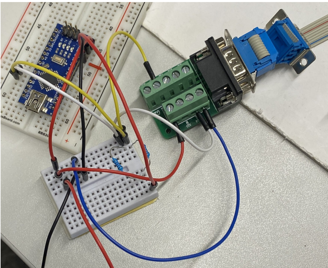
Abbildung 2: Verschaltung mit ATmega328P
