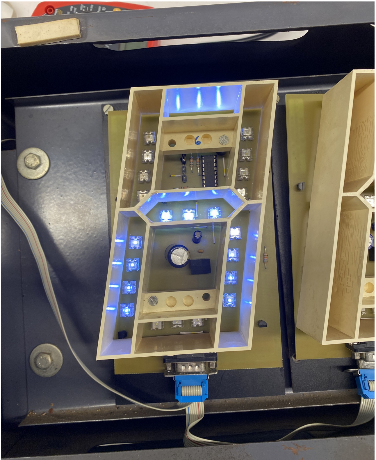
Abbildung 3: Test einer Anzeige
