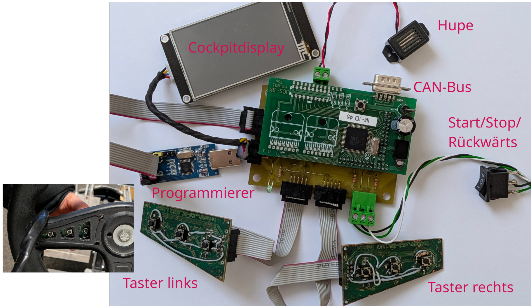
Abbildung 2: Cockpitplatine mit allen Geräten angeschlossen
