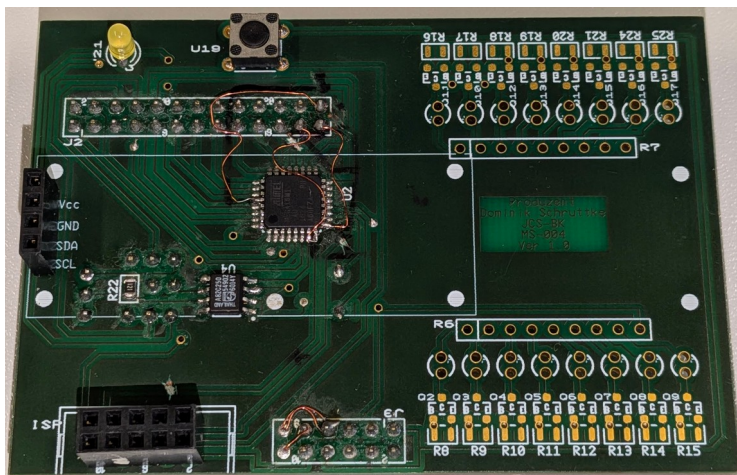
Abbildung 10: Oberseite des ATmega16M1
