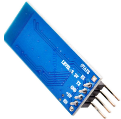
Abbildung 21: Bluetooth-Modul mit HC-06 Unterseite (Quelle: roboter-bausatz.de)
