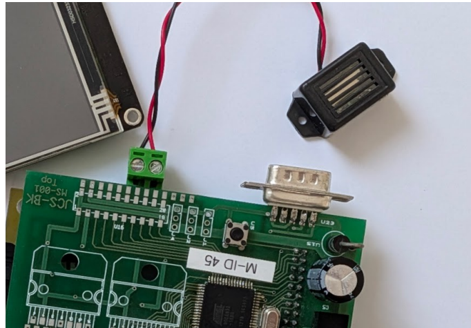
Abbildung 23: Miniatur Summer 24V (EMS-24L)
