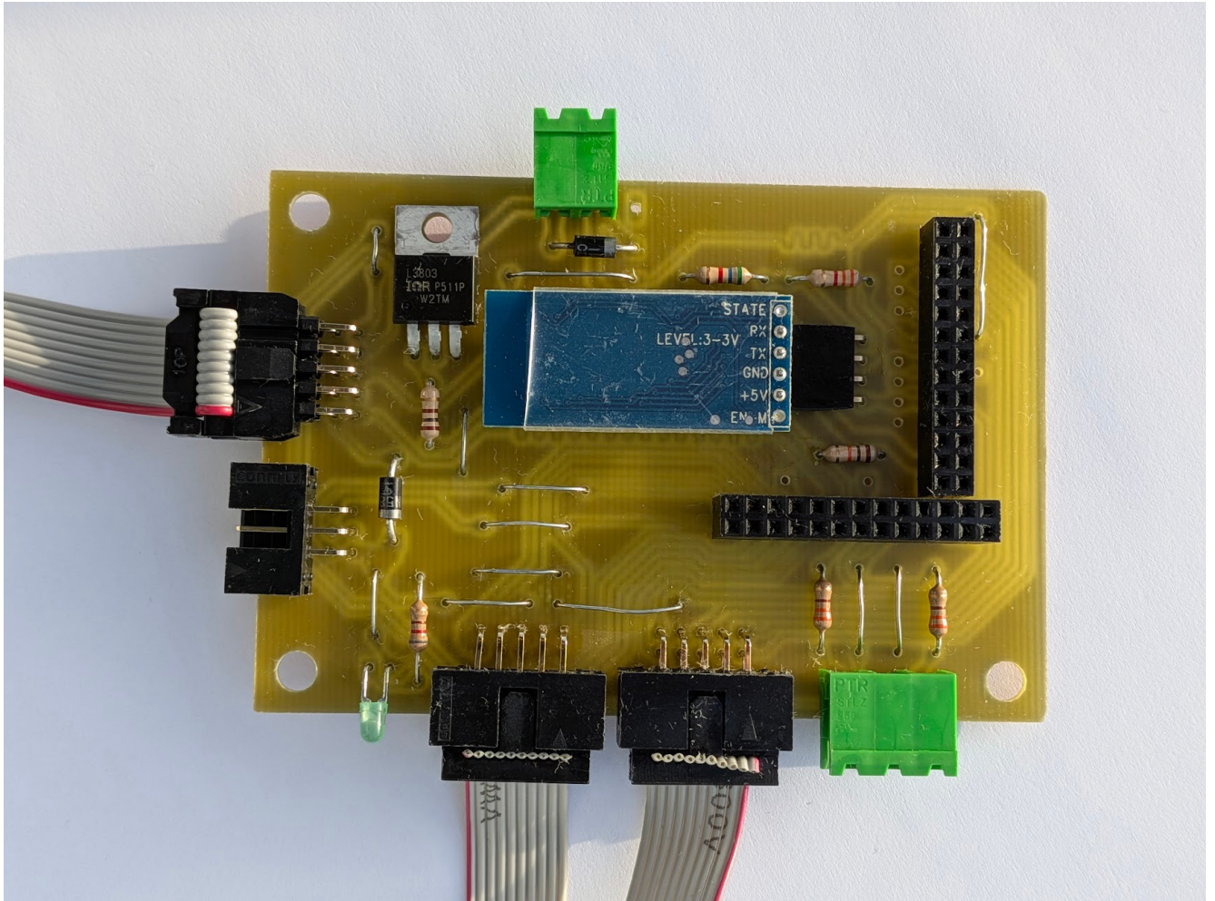
Abbildung 6: Bluetooth-Modul auf der Cockpitplatine
