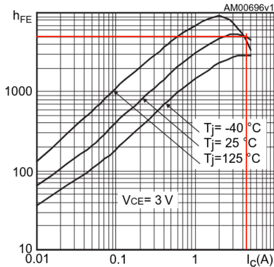
Abbildung 24: Kennlinien (Quelle: Datenblatt TIP120)
