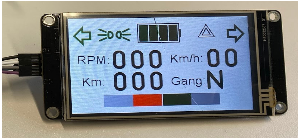
Abbildung 19: Cockpit-Display (NX4024K032)
