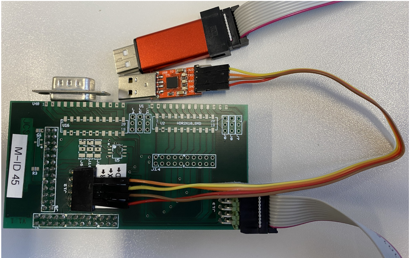
Abbildung 15: Masterplatine mit serieller und ISP Verbindung
