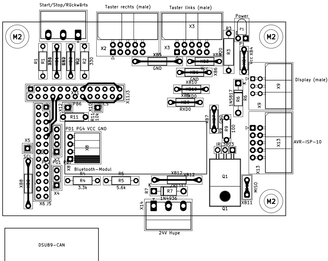
Abbildung 4: Bauteilansicht (top) der Cockpitplatine Rev 2
