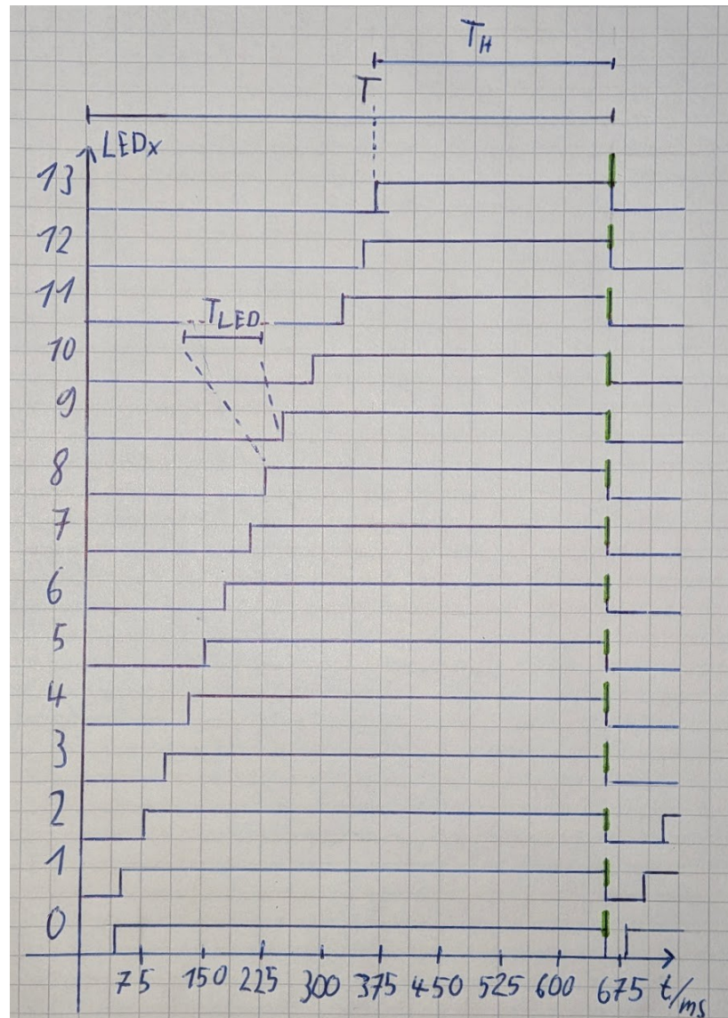
Abbildung 16: Signalzeitdiagramm der Blinker LEDs
