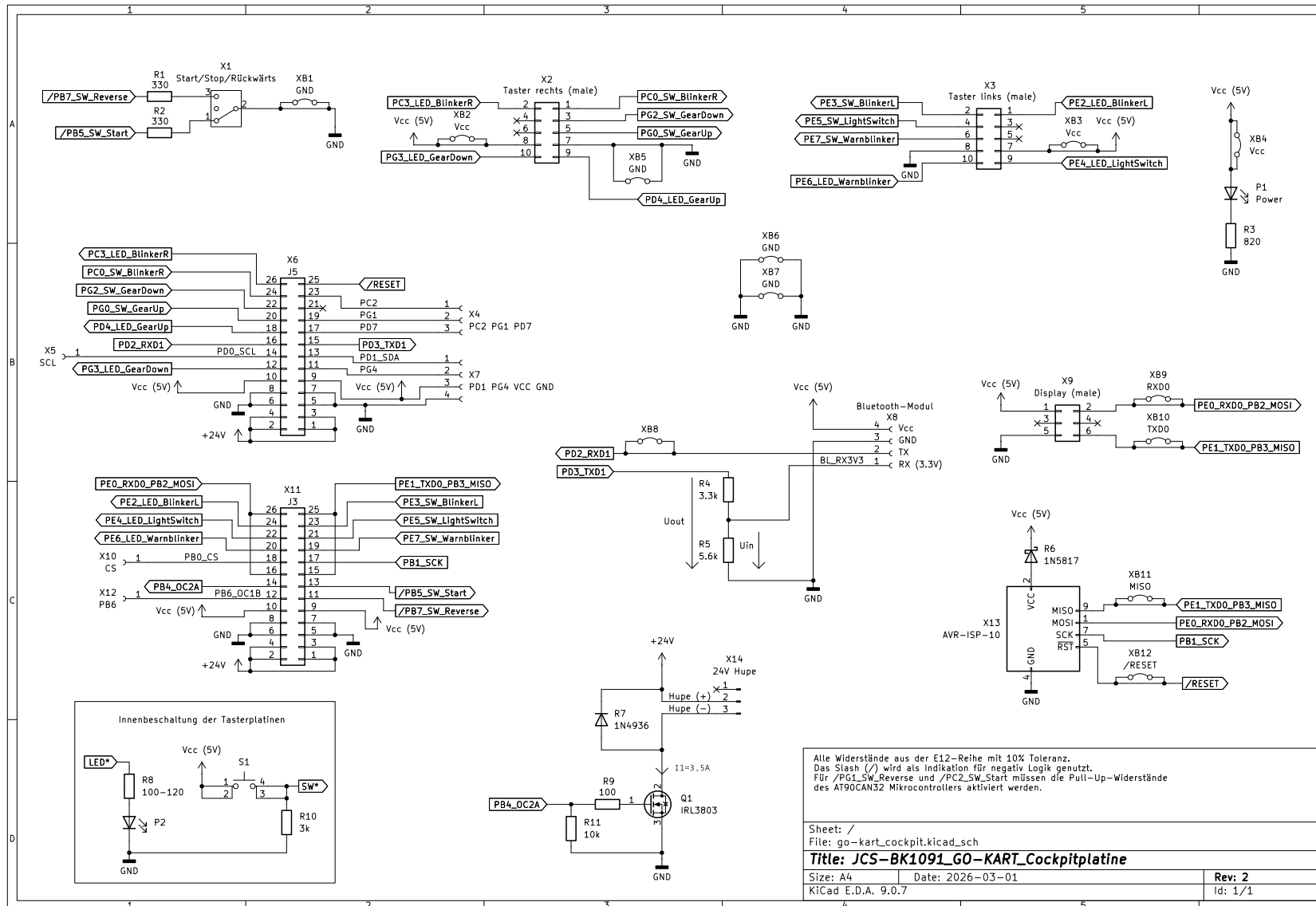
Abbildung 3: Schaltplan der Cockpitplatine Rev 2
