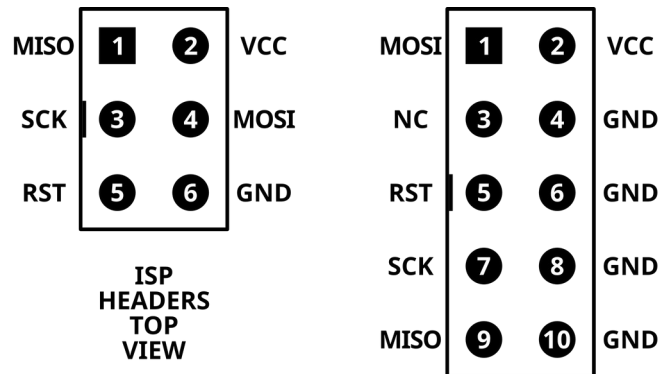
Abbildung 14: ISP Pinbelegung (Quelle: wikipedia.org von osiixy erstellt)
