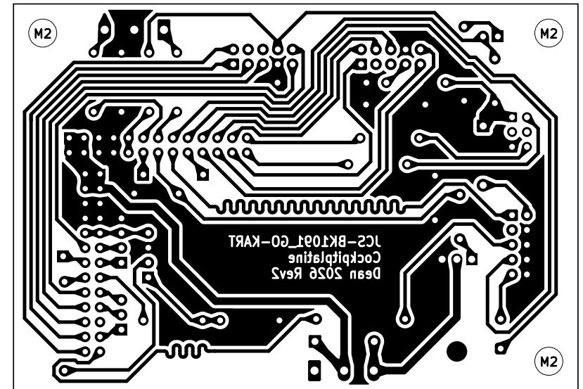
Abbildung 5: Leiterbahnen (bottom) der Cockpitplatine Rev 2
