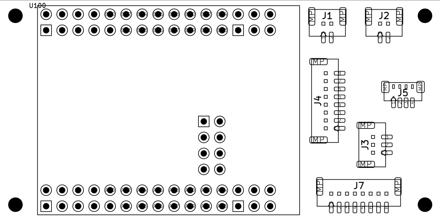
正面装配图
