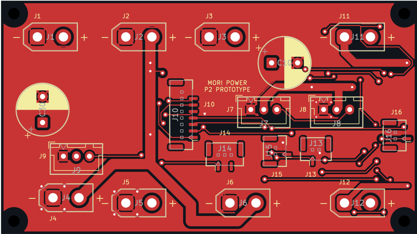
正面装配图
