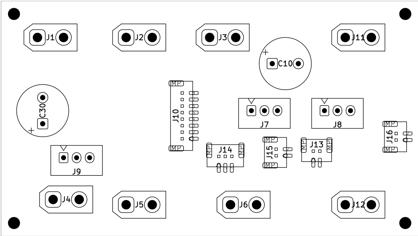
正面装配图
