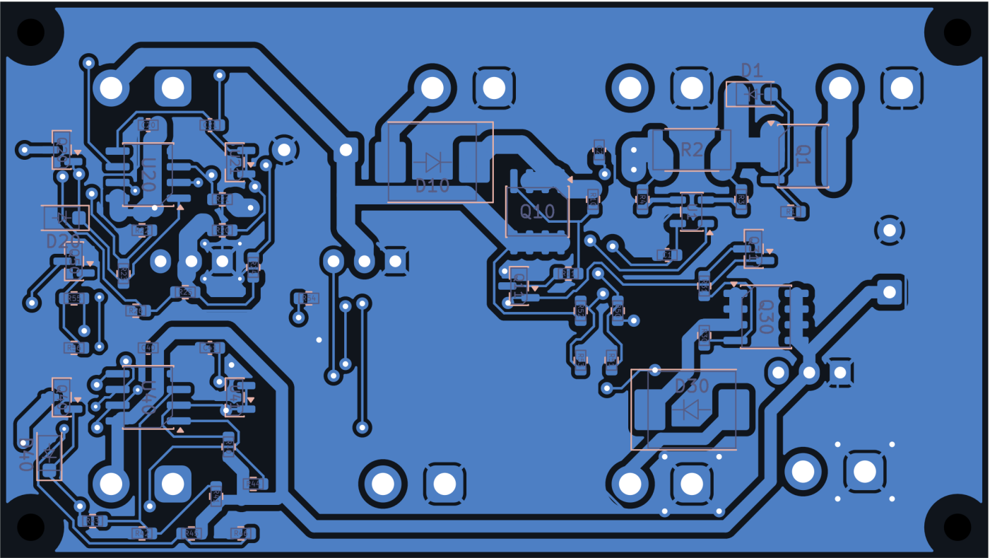
背面装配图 (已镜像)
