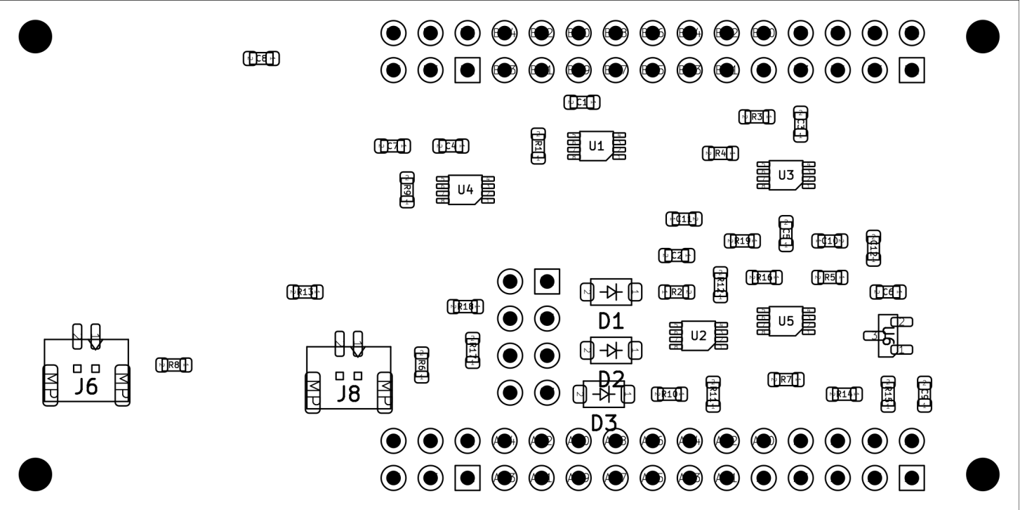
背面装配图 ( 已镜像 )
