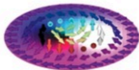
Bimeron
