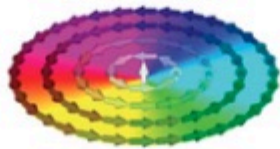
Vortex
