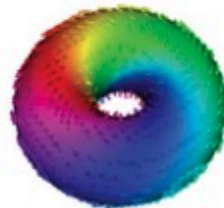
Hopfion
