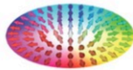
Meron
