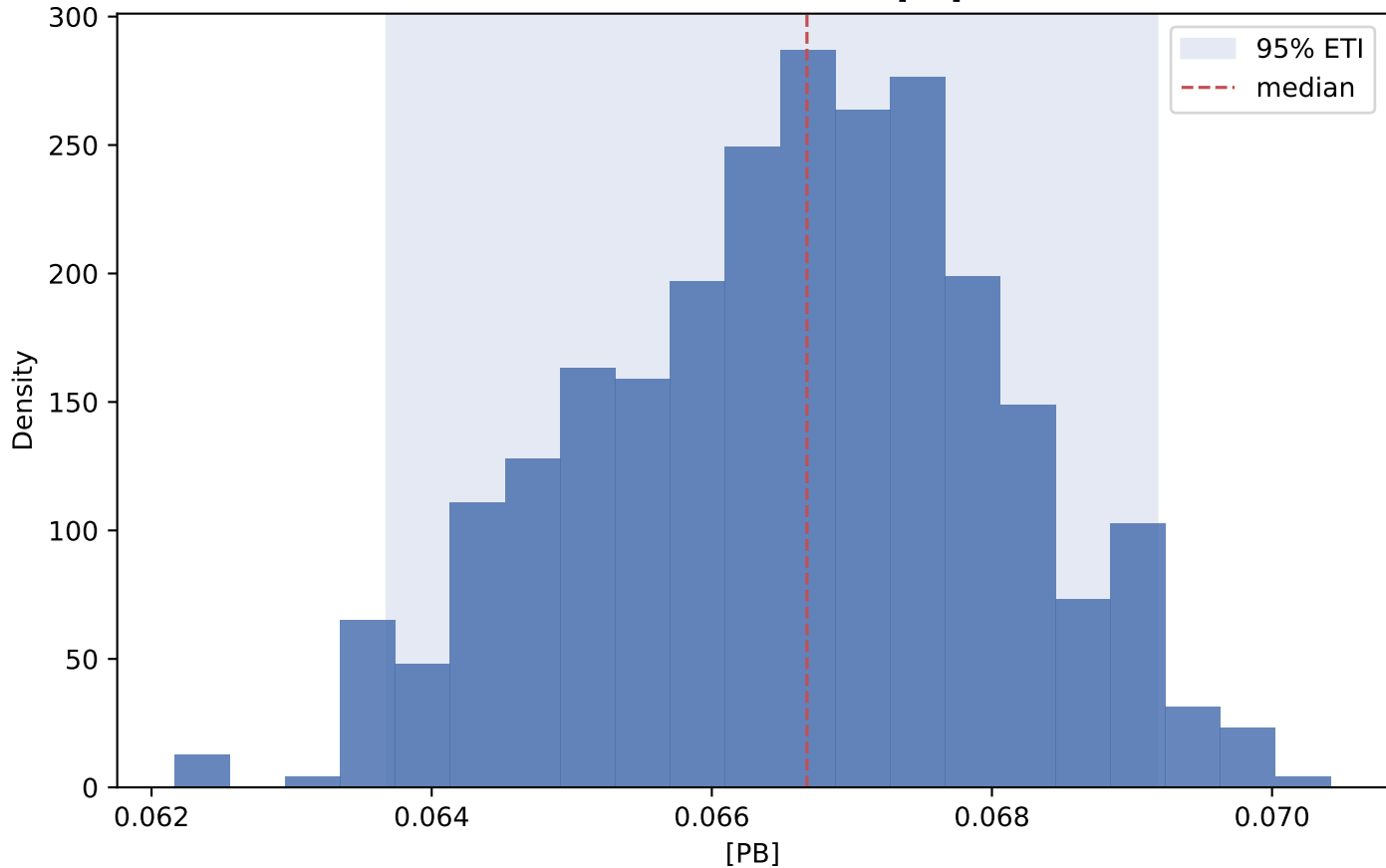
Posterior distribution: [PB]
