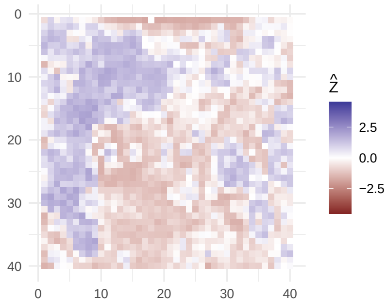
(d) Total fitted surface: \hat{Z}_k = X_k^T \hat{\beta} + \hat{u}_k
