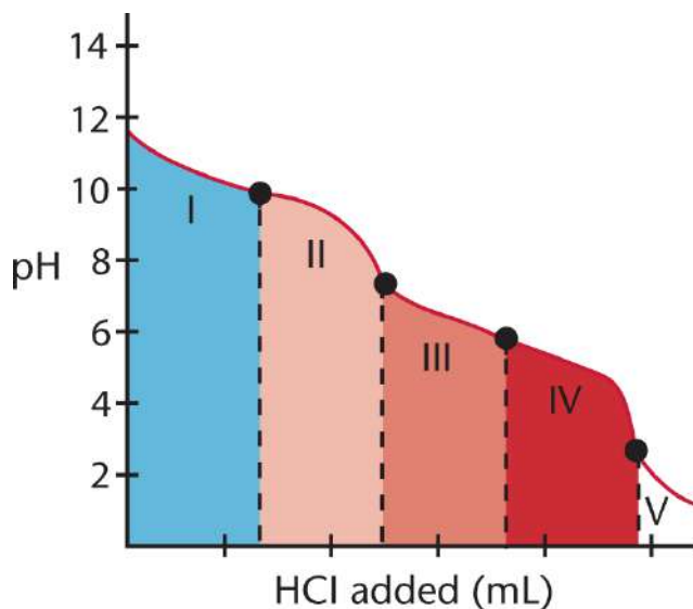
Figure 10.12. Polyvalent Titration
