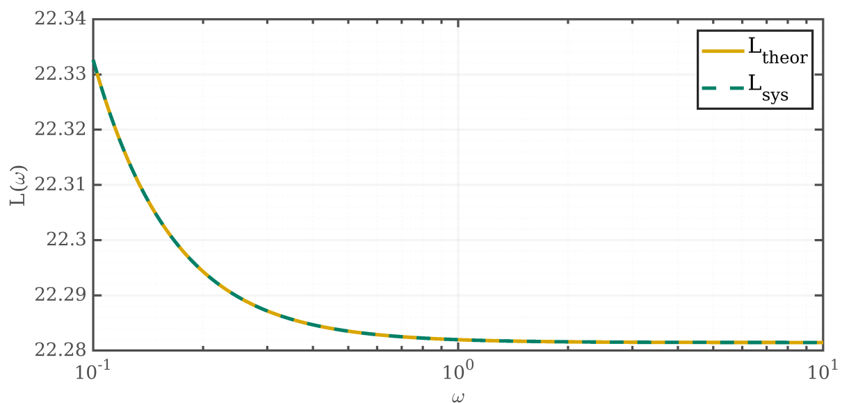
Рисунок 30: ЛАЧХ
