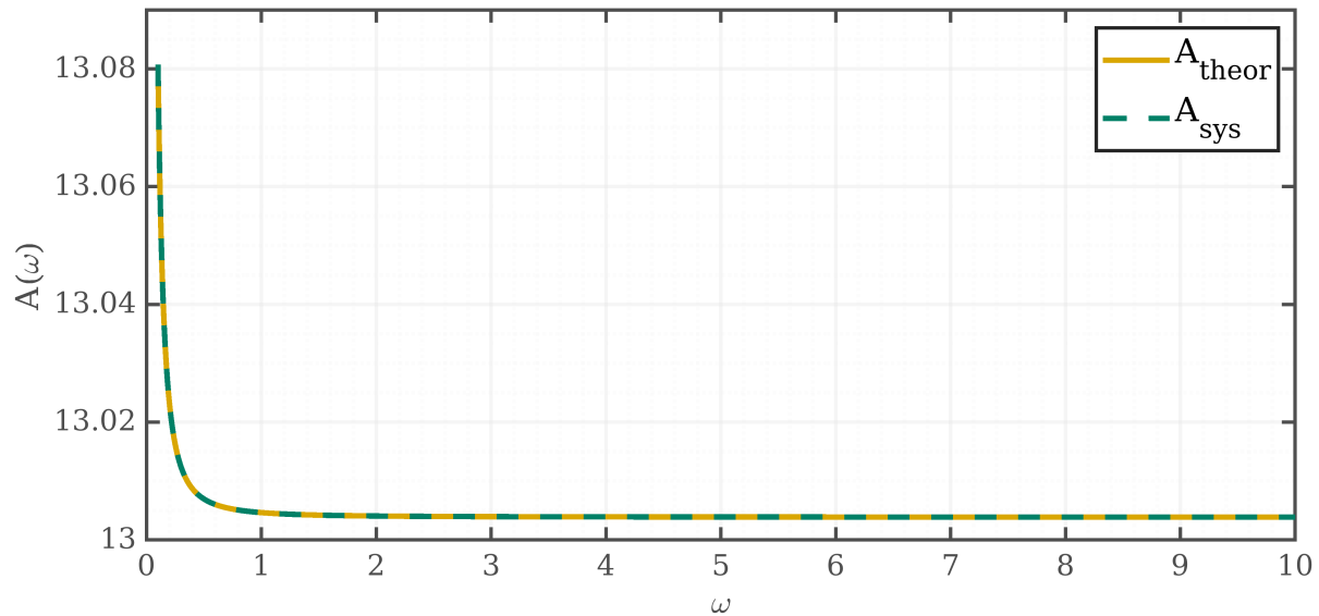
Рисунок 29: АЧХ
