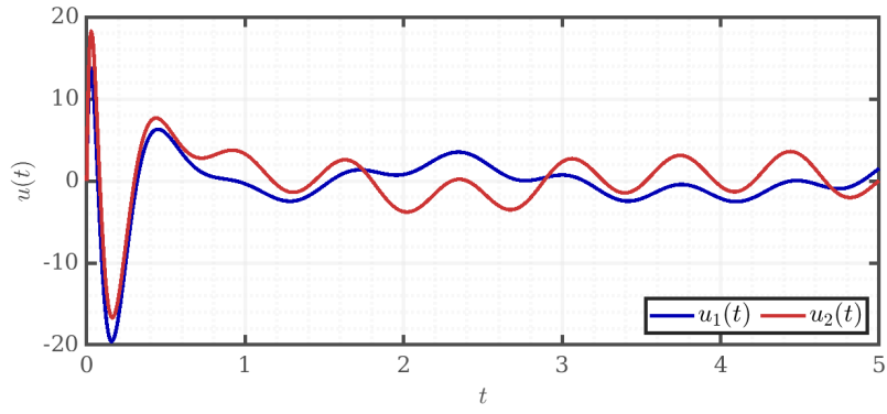
Рисунок 11 – Управление u(t)
