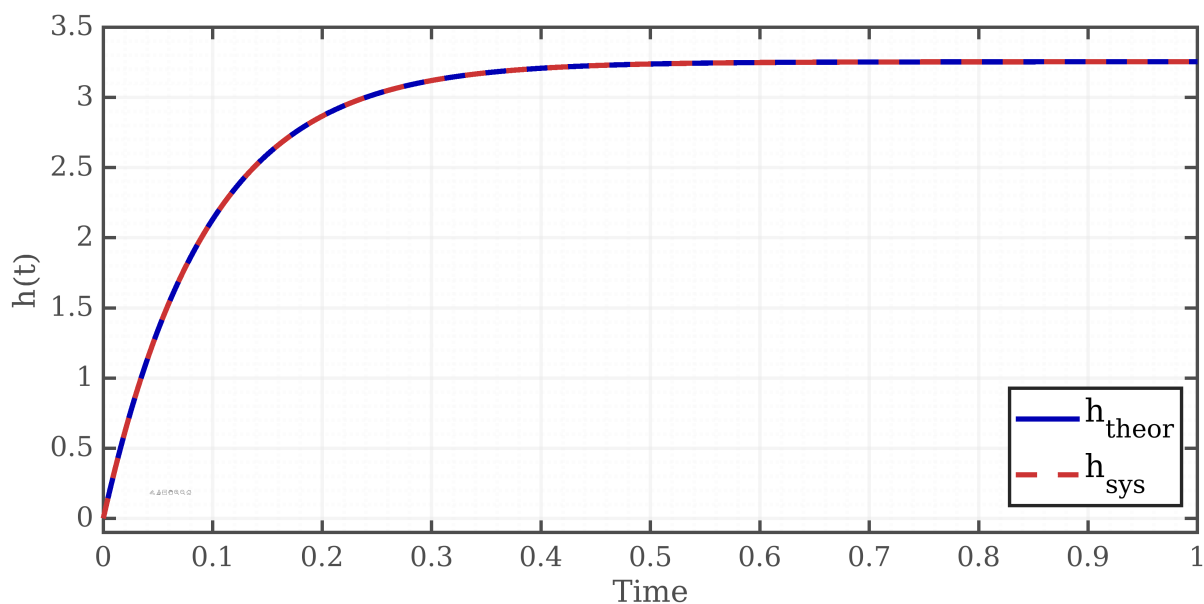
Рисунок 2: Переходная функция
