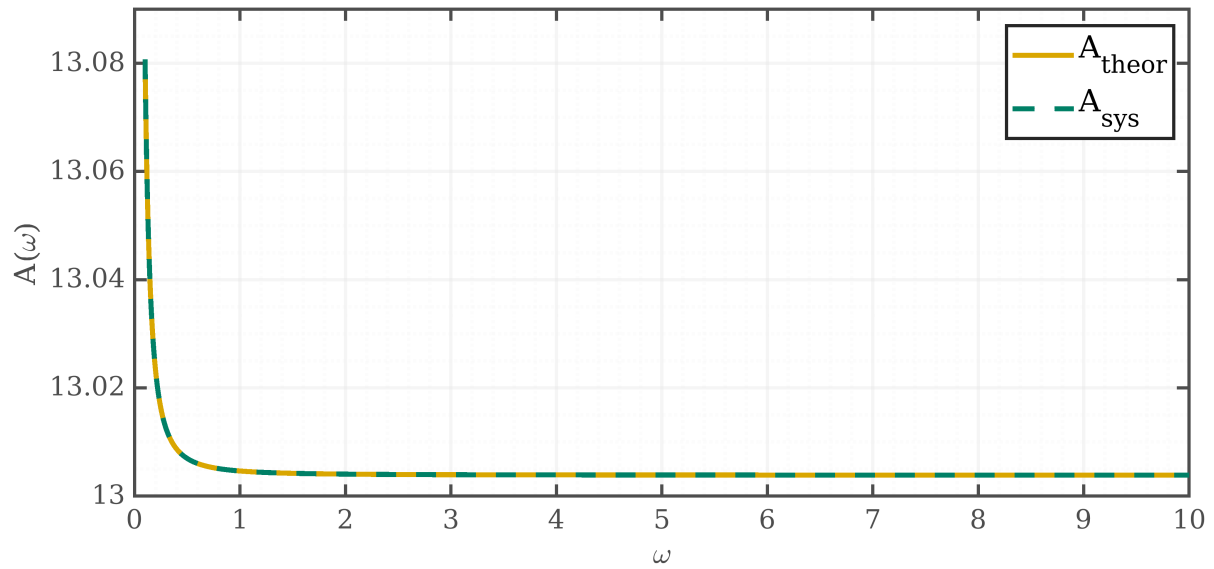
Рисунок 29: АЧХ
