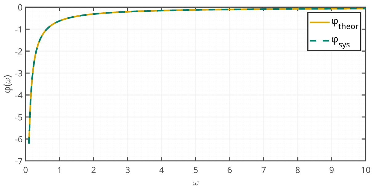
Рисунок 31: ФЧХ
