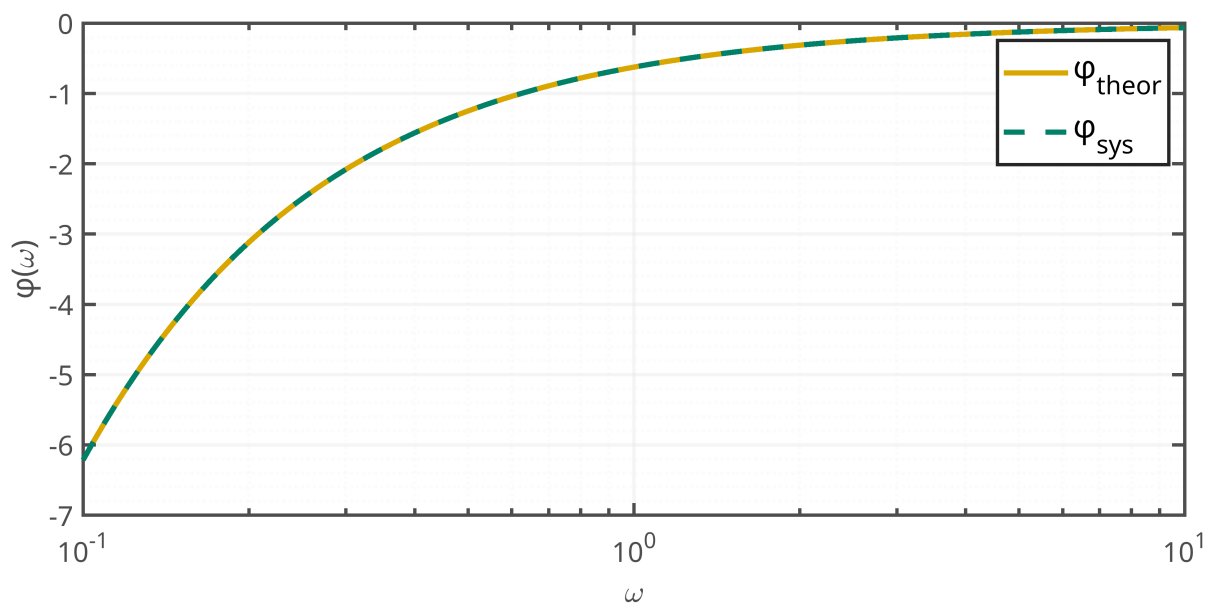
Рисунок 32: ЛФЧХ
