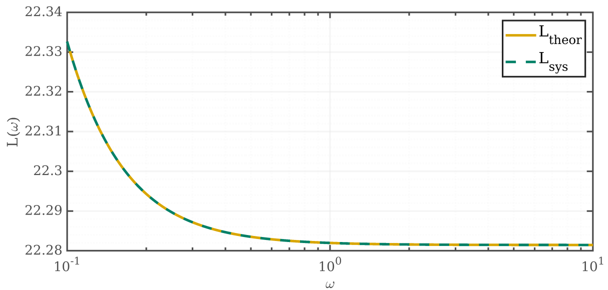
Рисунок 30: ЛАЧХ
