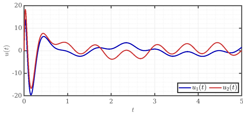
Рисунок 11 – Управление u(t)
