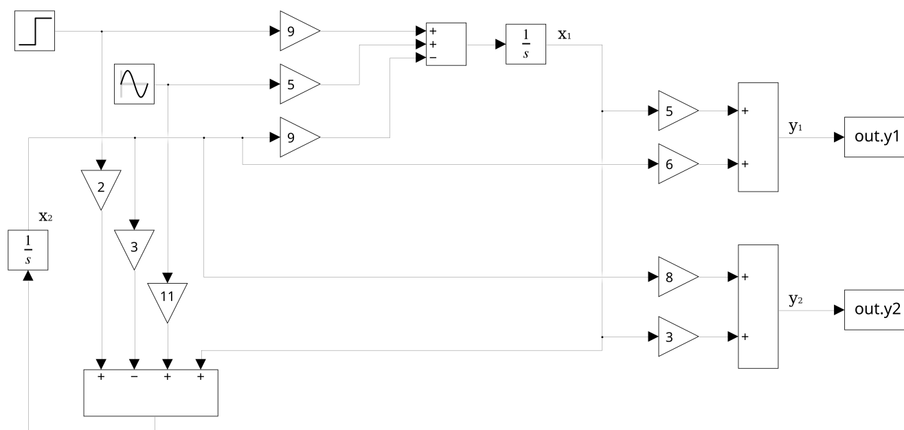
Рис. 13: Структурная схема многоканальной системы в форме В-С-В
