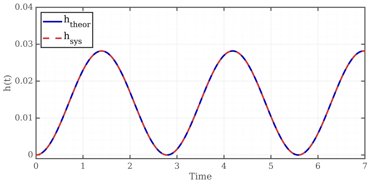
Рисунок 21: Переходная функция
