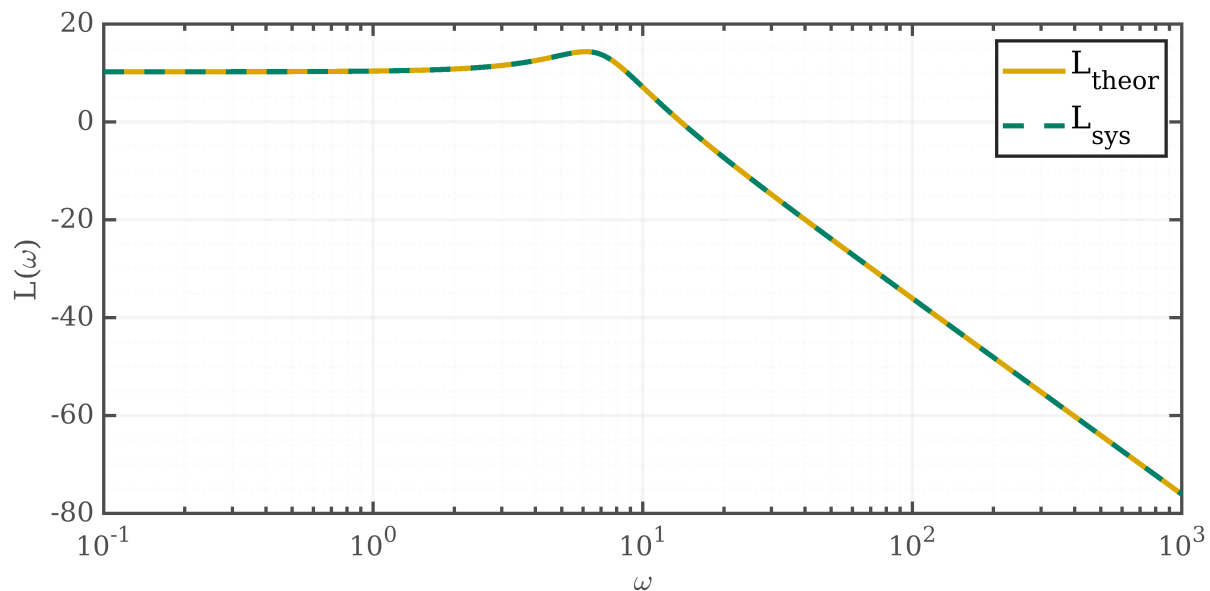
Рисунок 10: ЛАЧХ
