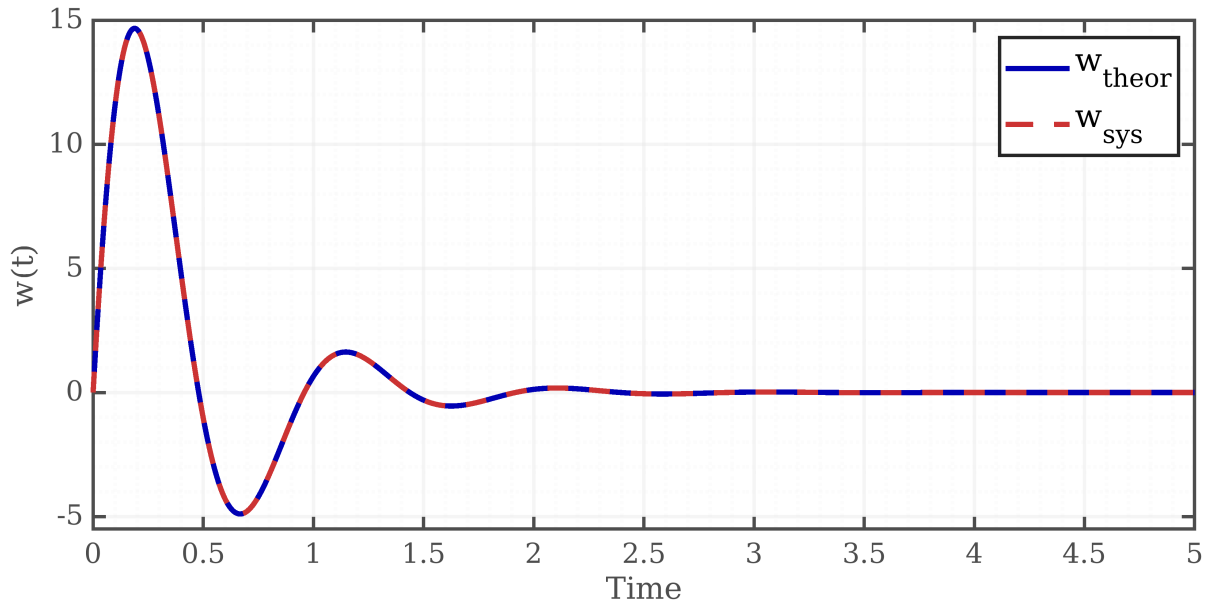
Рисунок 7: Весовая функция
