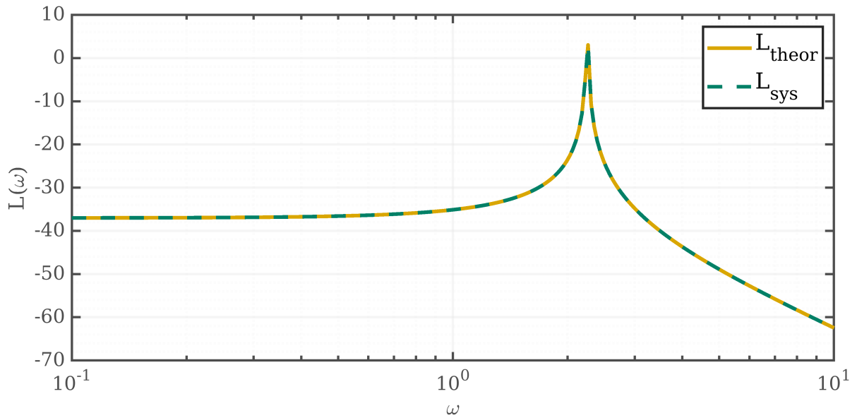
Рисунок 23: ЛАЧХ
