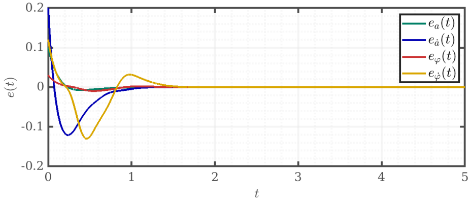
Рис. 97: Ошибки наблюдения e(t) = x(t) - \hat{x}(t)
