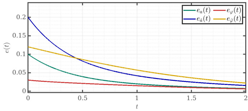
Рис. 61: Ошибки полного наблюдателя, медленный спектр
