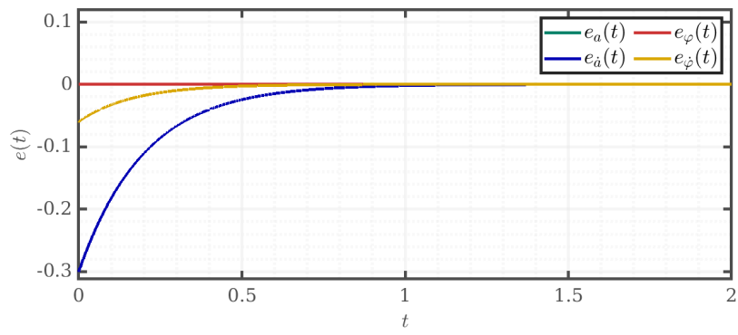
Рис. 68: Ошибки пониженного наблюдателя, средний спектр
