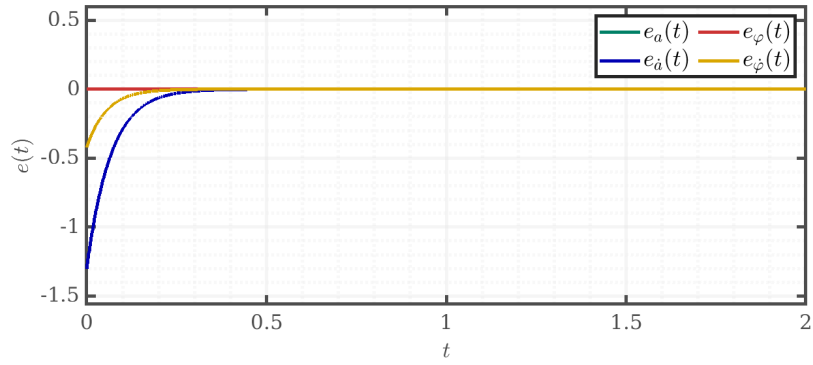
Рис. 69: Ошибки пониженного наблюдателя, быстрый спектр
