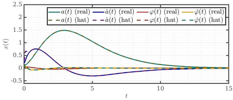
Рис. 66: Сравнение состояния и оценки, полный наблюдатель, быстрый спектр
