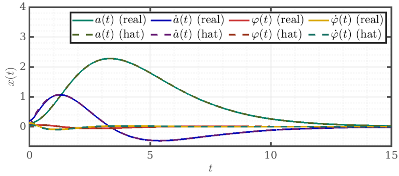
Рис. 65: Сравнение состояния и оценки, полный наблюдатель, средний спектр
