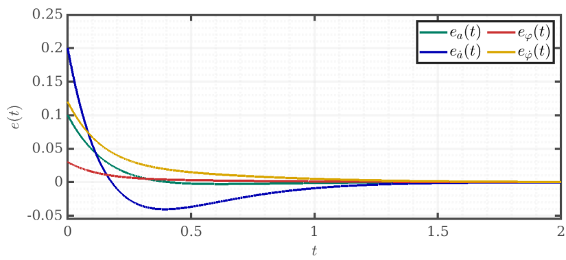
Рис. 62: Ошибки полного наблюдателя, средний спектр
