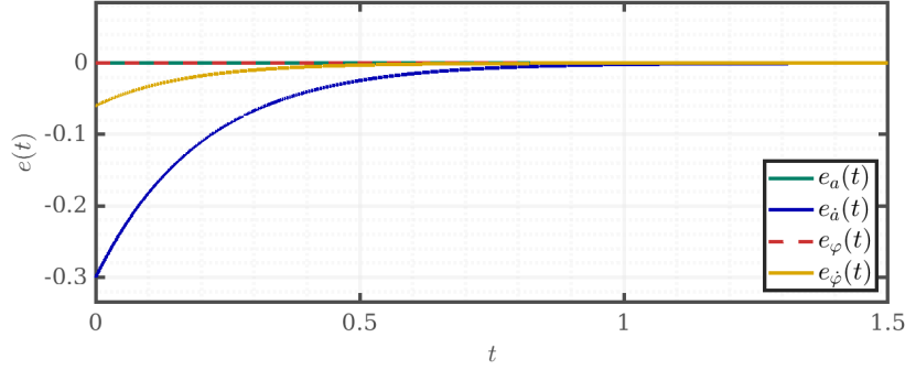
Рис. 59: Ошибки наблюдения пониженного наблюдателя
