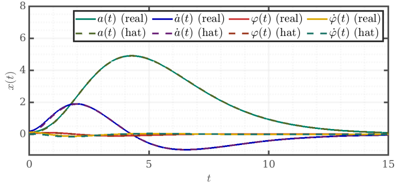
Рис. 64: Сравнение состояния и оценки, полный наблюдатель, медленный спектр
