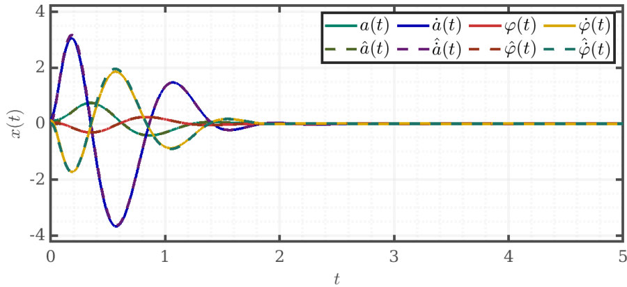
Рис. 98: Сравнение реального состояния x(t) и его оценки \hat{x}(t)
