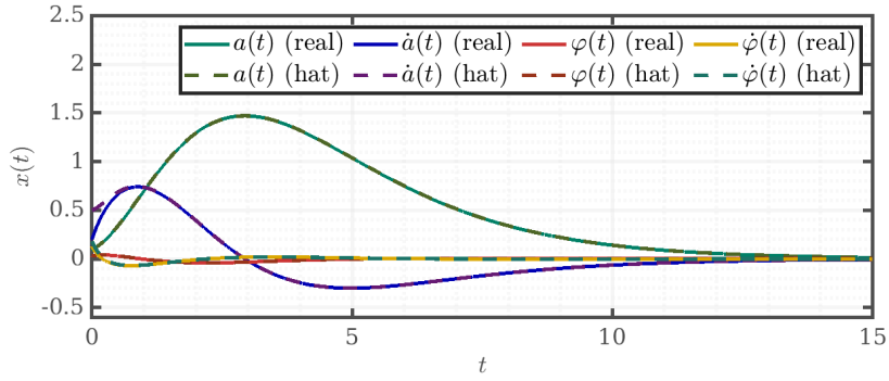
Рис. 71: Сравнение состояния и оценки, пониженный наблюдатель, средний спектр
