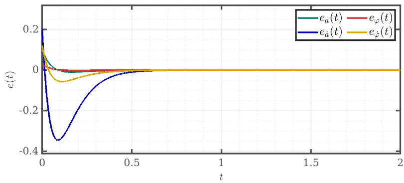
Рис. 63: Ошибки полного наблюдателя, быстрый спектр
