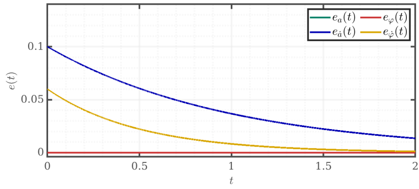
Рис. 67: Ошибки пониженного наблюдателя, медленный спектр
