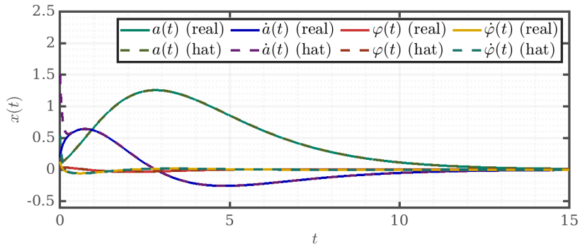
Рис. 72: Сравнение состояния и оценки, пониженный наблюдатель, быстрый спектр
