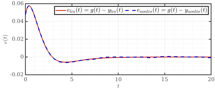
Рис. 122: Ошибка слежения e(t) = g(t) - \varphi(t) , успешный случай
