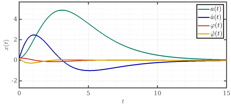
Рис. 48: x(0) = [0.2, 0.2, 0.2, 0.2]^T — успешный
