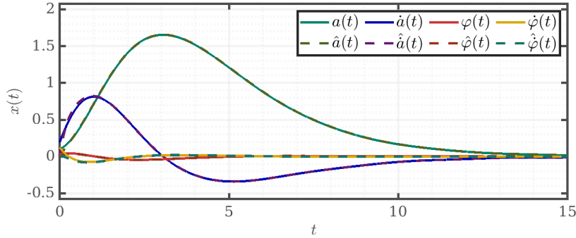
Рис. 57: Сравнение реального состояния x(t) и его оценки \hat{x}(t)
