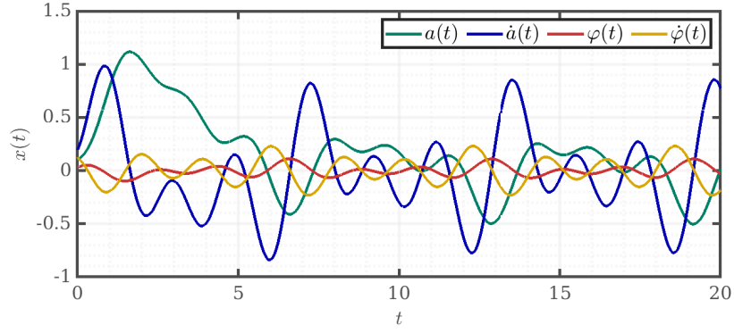
Рис. 120: Нелинейная модель, успешное слежение
