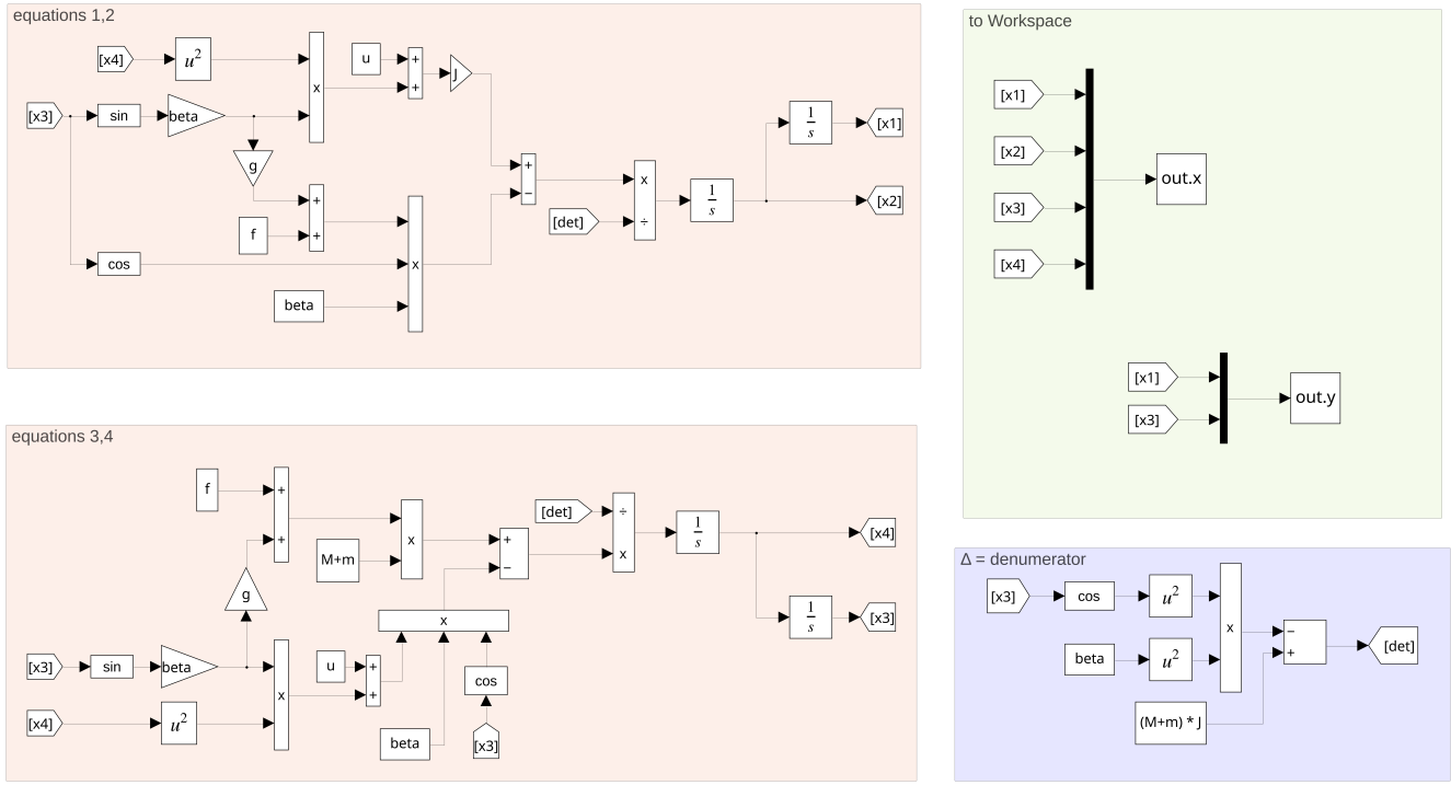
Рис. 2: Структурная схема нелинейной системы
