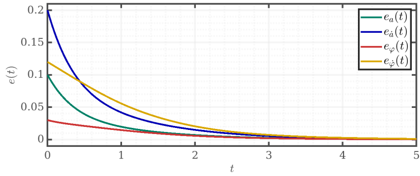
Рис. 76: Ошибки наблюдения, равные спектры)
