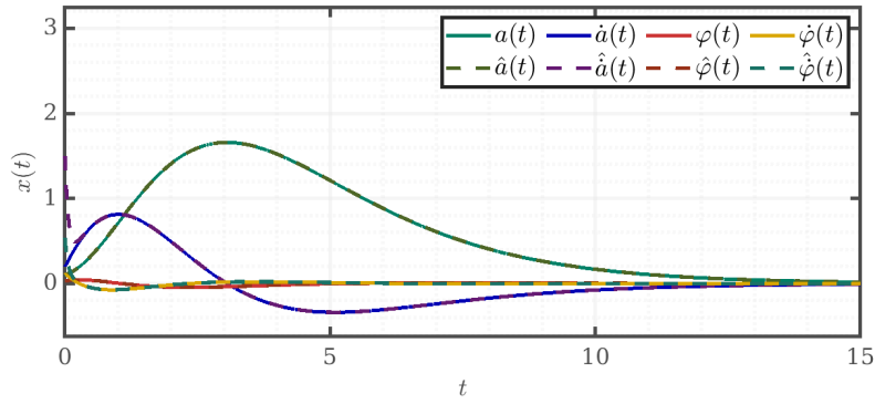
Рис. 72: Сравнение состояния и оценки, пониженный наблюдатель, быстрый спектр
