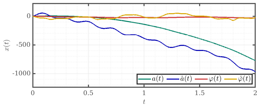
Рис. 124: Нелинейная модель, неуспешное слежение
