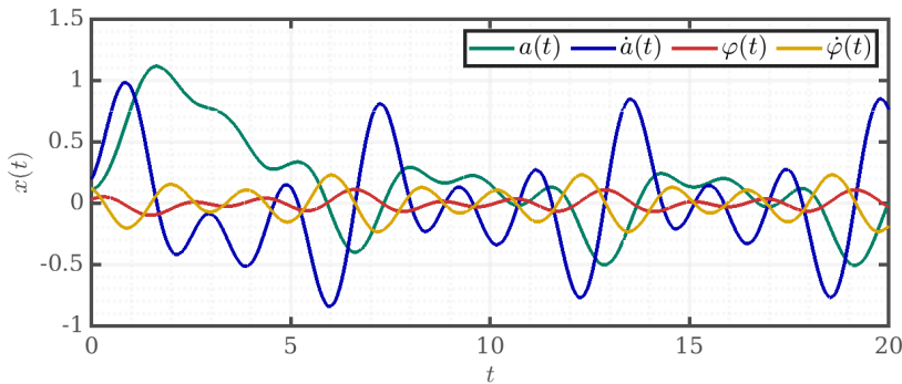
Рис. 119: Линейная модель, успешное слежение
