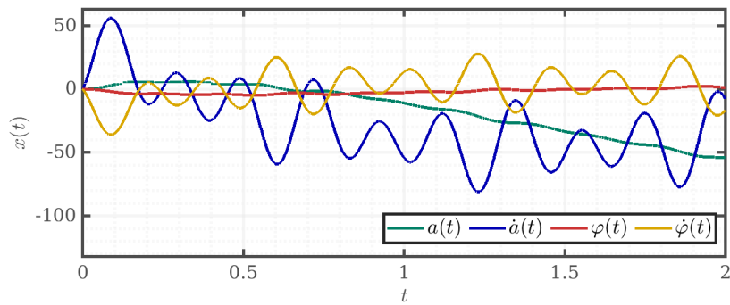
Рис. 123: Линейная модель, неуспешное слежение
