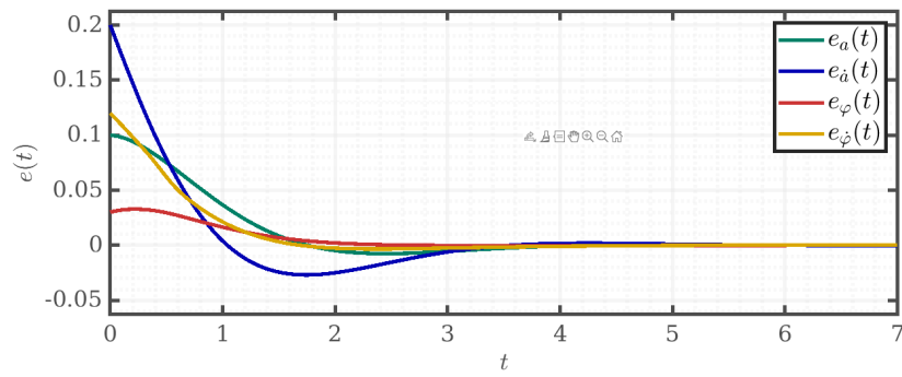
Рис. 109: Ошибки наблюдения, \alpha = 3, \beta = 0.5 — сильный регулятор + медленный наблюдатель
