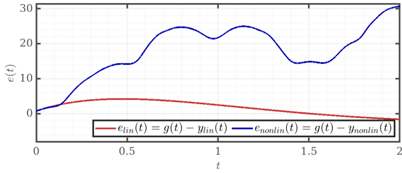
Рис. 126: Ошибка слежения e(t) = g(t) - \varphi(t) , неуспешный случай
