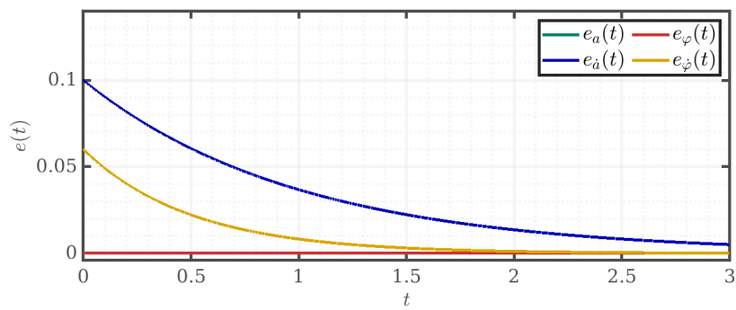
Рис. 67: Ошибки пониженного наблюдателя, медленный спектр
