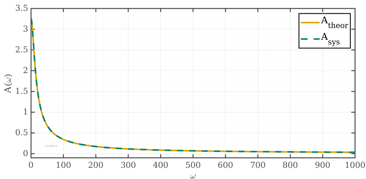
Рисунок 3: АЧХ
