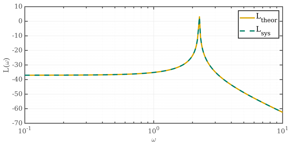
Рисунок 23: ЛАЧХ
