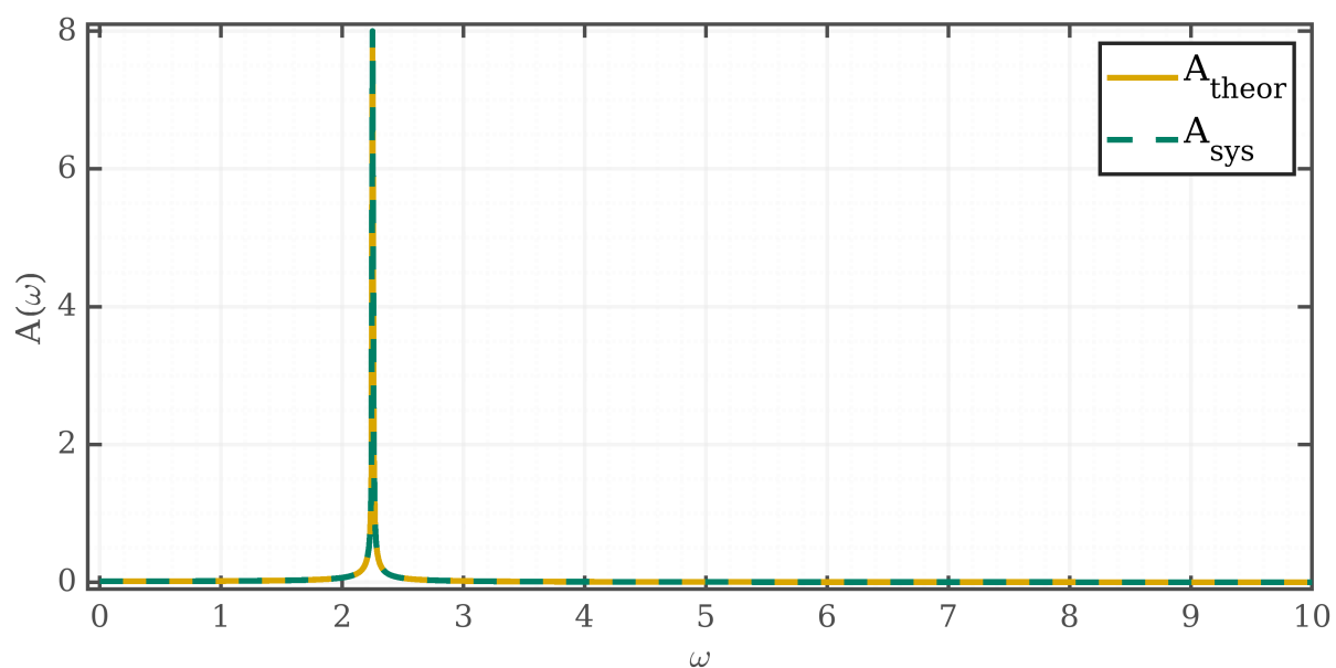
Рисунок 22: АЧХ
