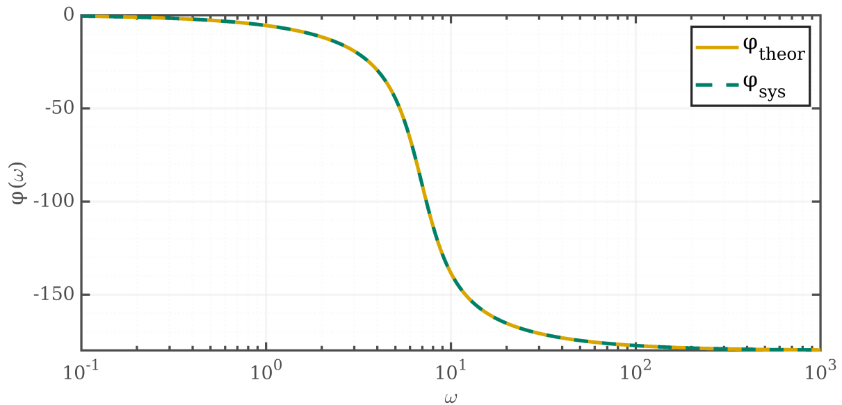
Рисунок 12: ЛФЧХ
