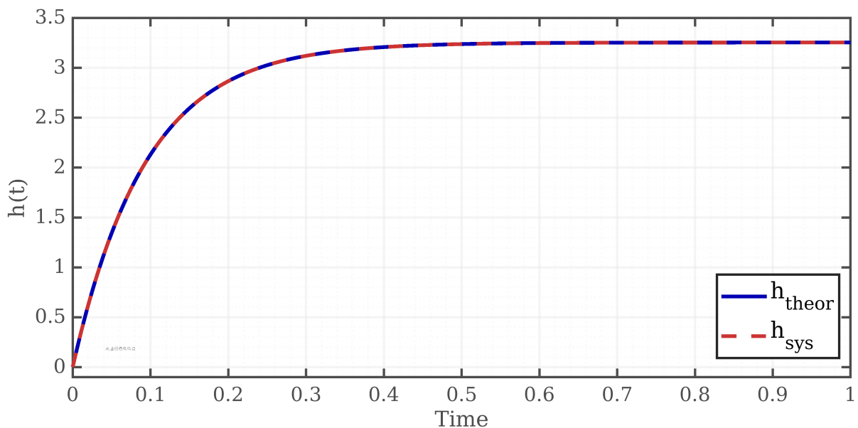
Рисунок 2: Переходная функция
