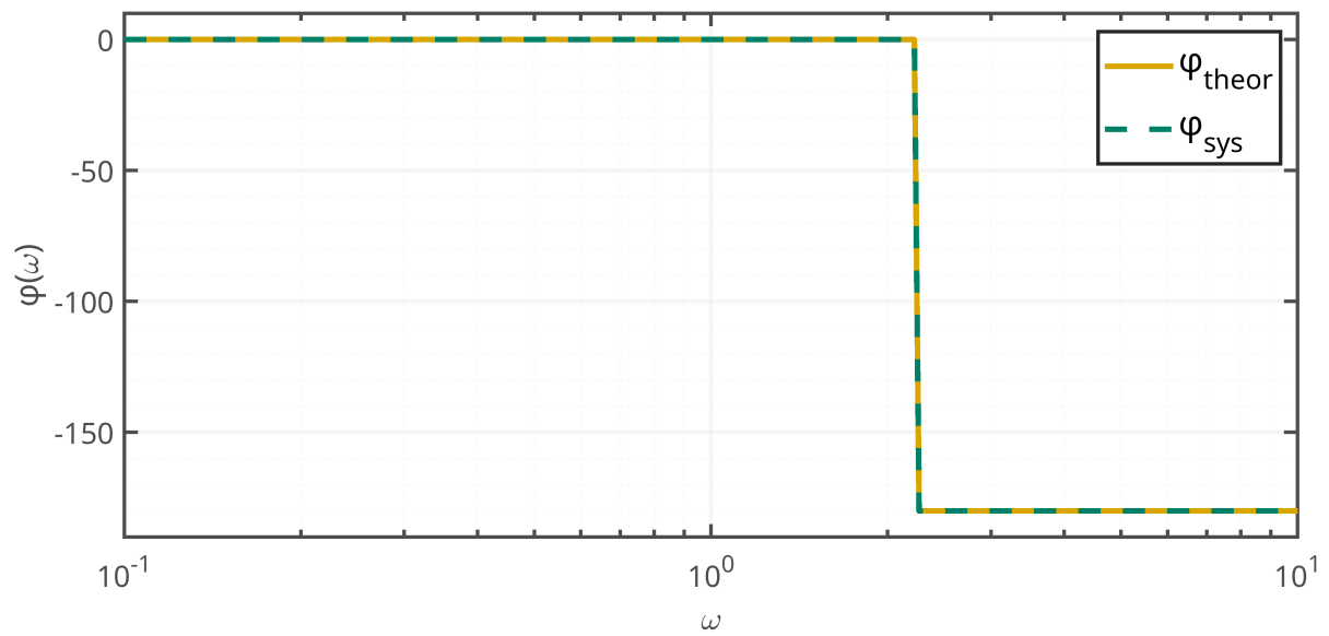
Рисунок 25: ЛФЧХ
