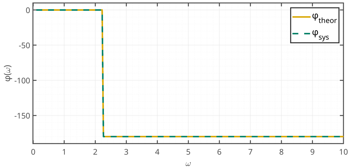
Рисунок 24: ФЧХ
