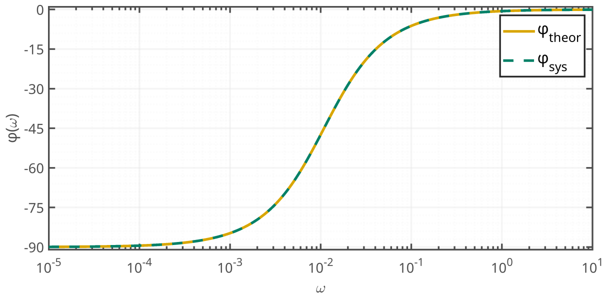
Рисунок 32: ЛФЧХ 1
