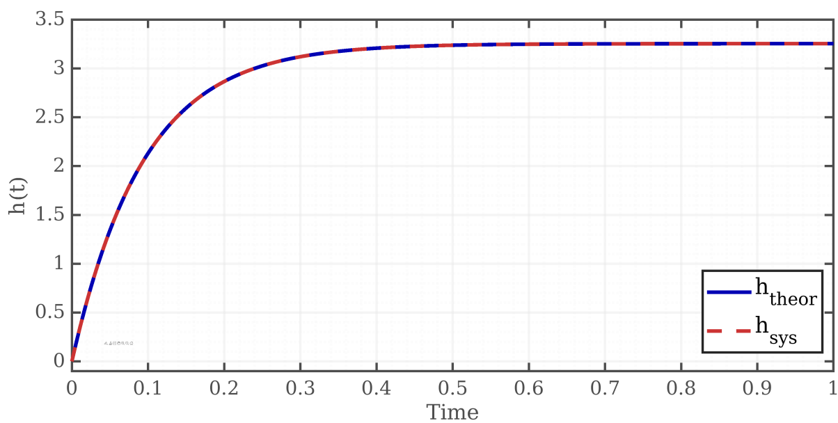
Рисунок 2: Переходная функция
