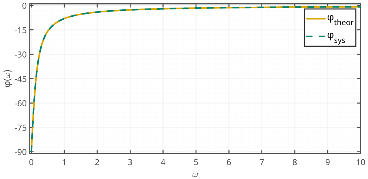
Рисунок 31: ФЧХ 1
