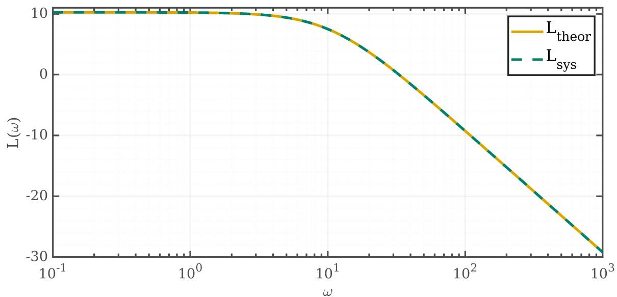
Рисунок 4: ЛАЧХ
