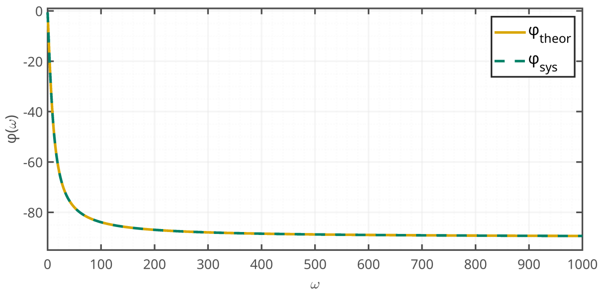
Рисунок 5: ФЧХ
