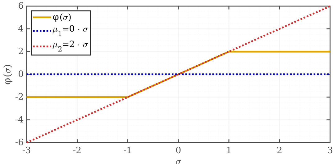
Рисунок 3: Выполнение секторного условия
