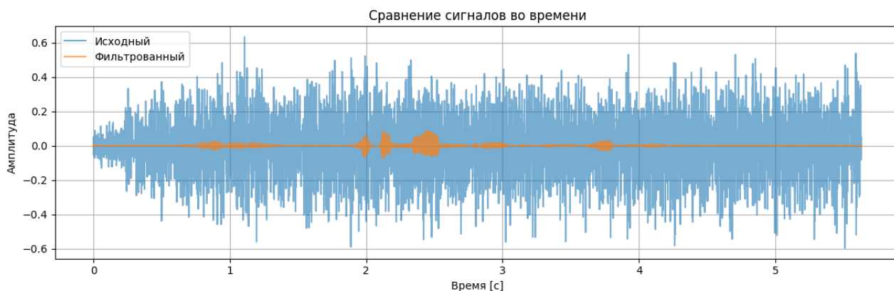
Рис. 26: График сигналов
