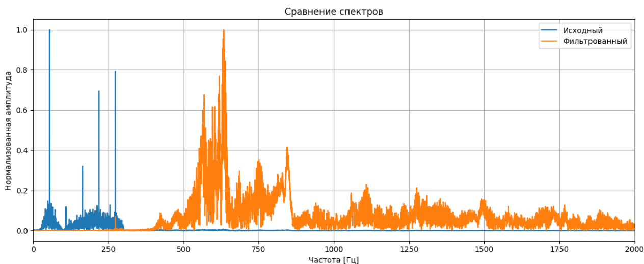
Рис. 27: График спектра
